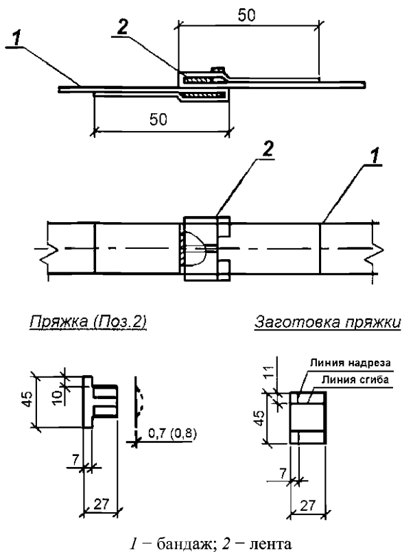
Рисунок 6.2 – Конструкция бандажа
