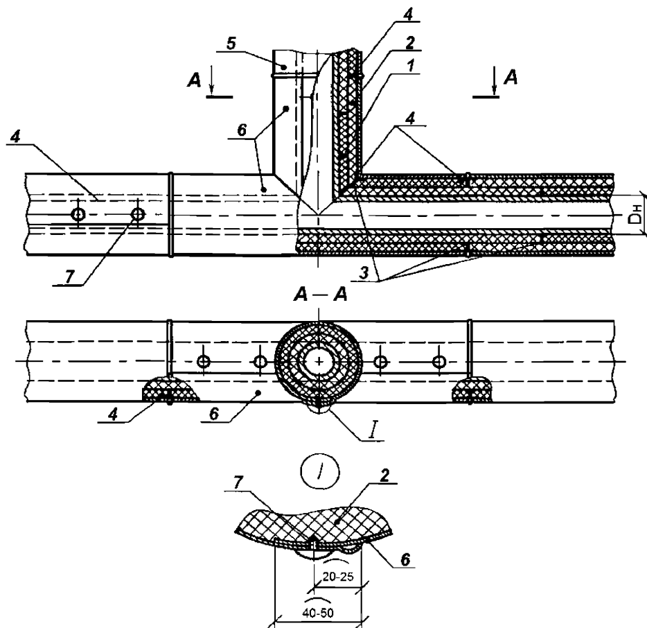
I – трубка из теплоизоляционного материала; 2 – лист теплоизоляционного материала; 3 – клей; 4 – лента армированная самоклеящаяся; 5, 6 – металлические оболочки; 7 – саморез с прессшайбой, оцинкованный, наконечник сверло Рисунок 6.5 – Теплоизоляционная конструкция тройника
