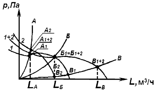
Рисунок 9.5 – Параллельная работа двух вентиляторов в сети
