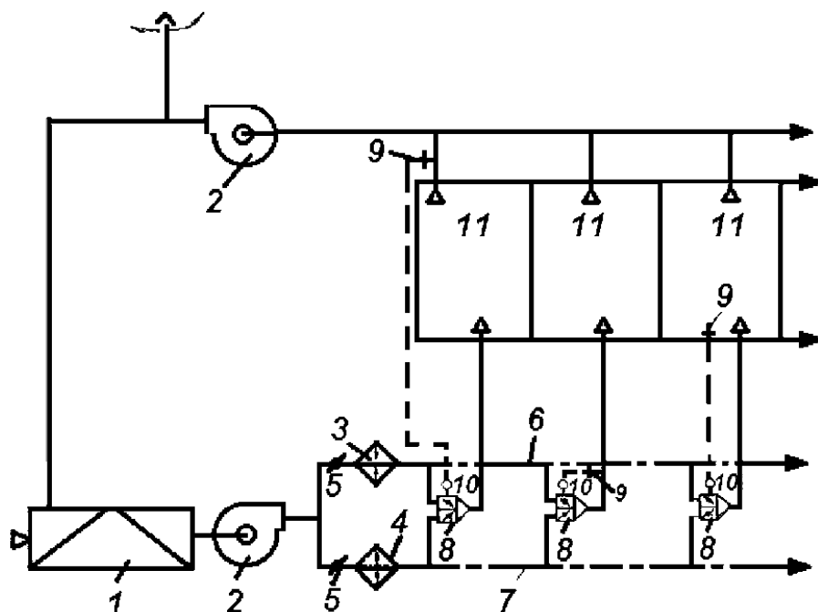
1 – кондиционер; 2 – вентилятор; 3 – воздушонагреватель; 4 – воздухоохладитель; 5 – воздушный клапан; 6 – коллектор теплого воздуха; 7 – коллектор холодного воздуха; 8 – смеситель; 9 – датчик терморегулятора; 10 – исполнительный механизм; 11 – кондиционируемое помещение
