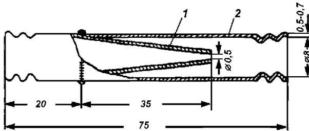
Рисунок 8.4 – Демпфер
