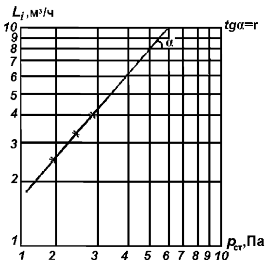
Рисунок 9.2 – График зависимости L_i = R (p_{\text{ст}})^r , полученный по результатам испытаний сетей воздухопроводов на герметичность, где R – коэффициент градуировки, равный расходу воздуха при p_{\text{ст}} = 1 Па
