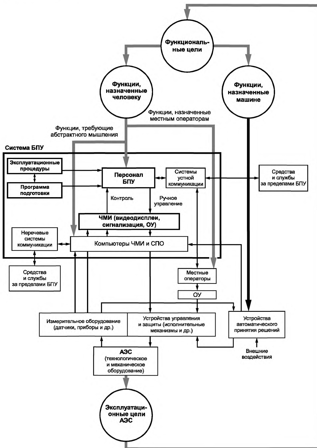
Рисунок 1 — Структура системы БПУ
