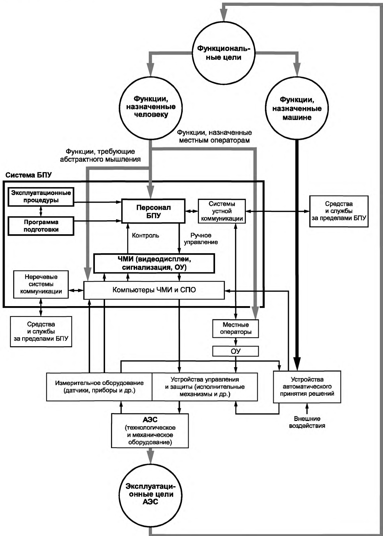
Рисунок 1 — Структура системы БПУ
