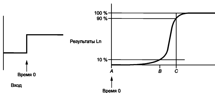
Рисунок 1 – Время срабатывания (чувствительность всей системы)
