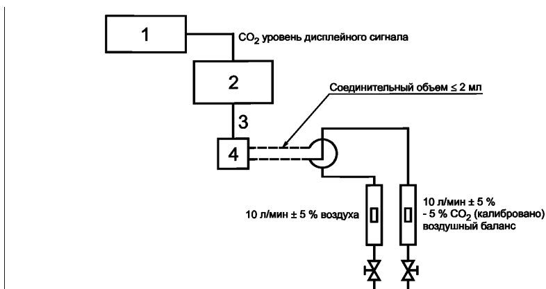
1 — самописец или осциллоскоп; 2 — капнометр; 3 — трубка образца; 4 — датчик или адаптер для трубки образца
