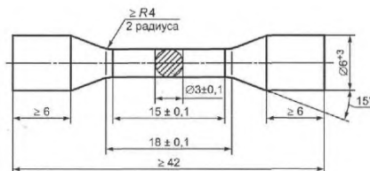
Рисунок 1 — Образец с короткой головкой
