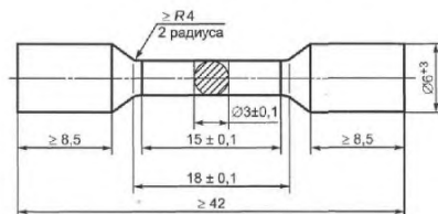
Рисунок 2 — Образец с удлиненной головкой
