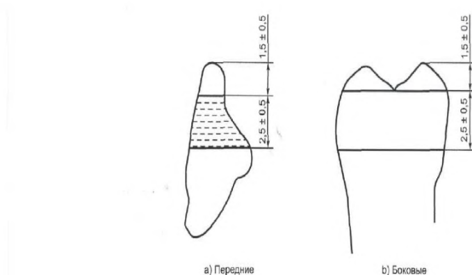
Рисунок 2 — Толщина образца зуба для испытания на пористость (см. 7.7)
