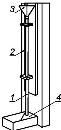
1 — стеклянная трубка; 2 — штатив; 3 — конусообразная воронка; 4 — ящик
