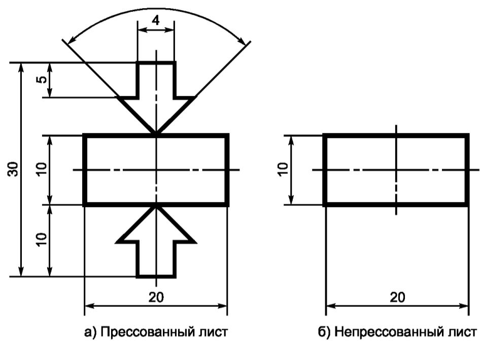
Рисунок Г.1 — Размеры символического изображения типа листов
