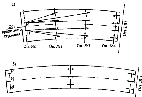
Рисунок 6 – Направление векторов перемещений для мостов, расположенных на кривых в плане
