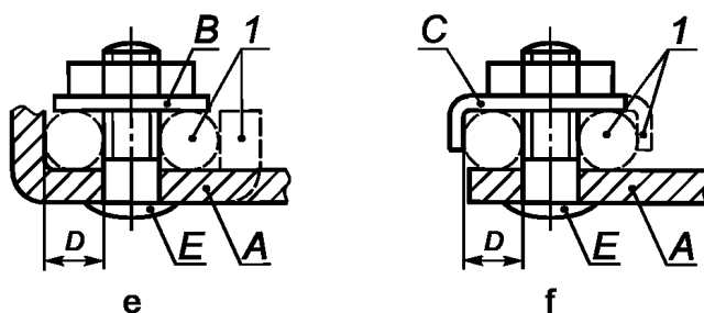
Зажимы с крепежной гайкой
