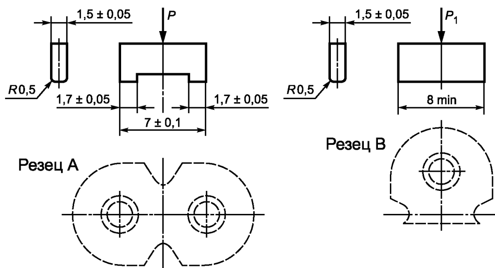
Рисунок 21 — Прибор для испытания на удар (ссылка — в 23.5)
