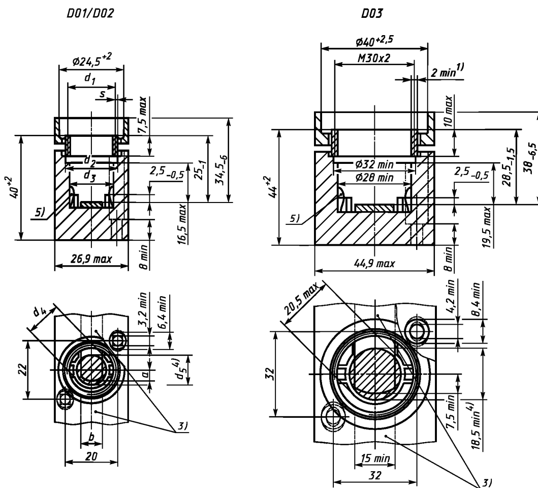
Рисунок 2 — Основные размеры оснований предохранителей типа D, лист 1
