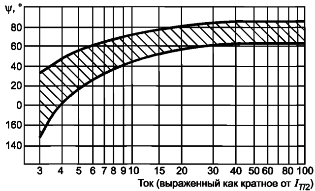
Рисунок 1 — Момент включения тока при испытании № 1
