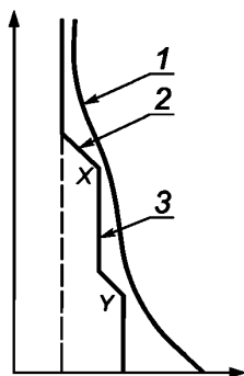
1 — преддуговая характеристика; 2 — прямая постоянного значения I^2t ; 3 — условная кривая перегрузок
