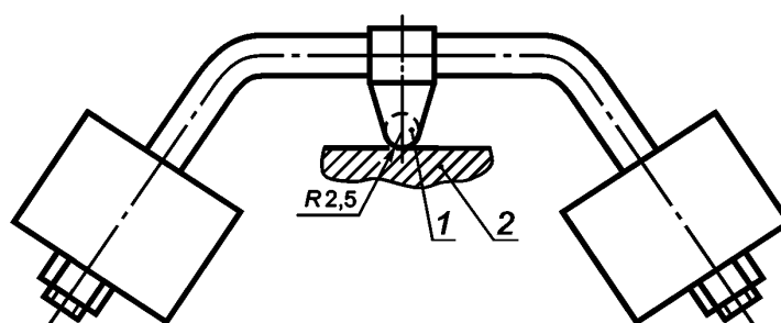
Установка для испытаний на твердость по Бринеллю
