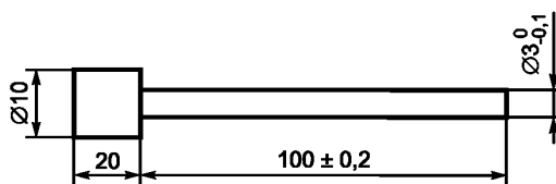
Рисунок 101— Испытательный стержень для скрытой блокировки
