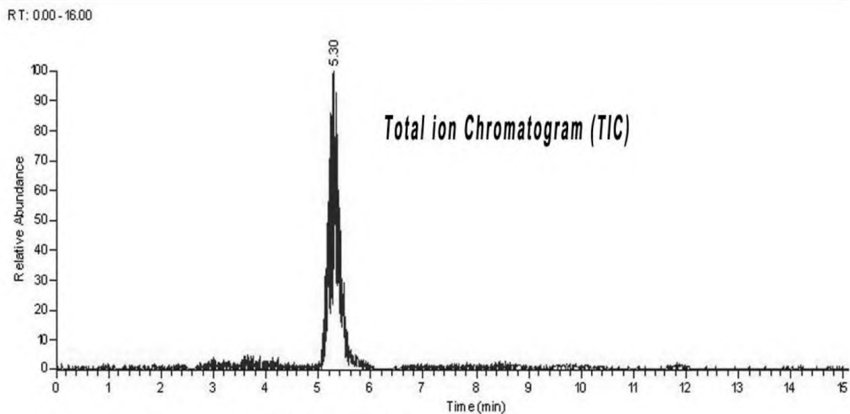
Рисунок В.1 — Хроматограмма LC-MS/MS меламина (MEL) из экстракта детской молочной смеси NIST при концентрации введенного вещества: MEL = 0,50 мг/кг
