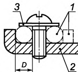
Зажимы, требующие применения прокладки, прижимной пластины или специальной прижимной детали
