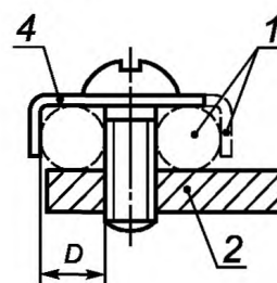
Зажимы, требующие применения прокладки, прижимной пластины или специальной прижимной детали
