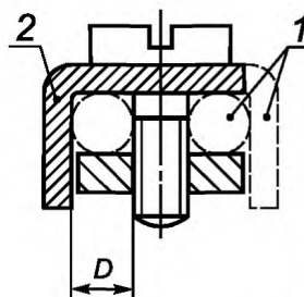
Зажимы, не требующие применения прокладки, прижимной пластины или специальной прижимной детали
