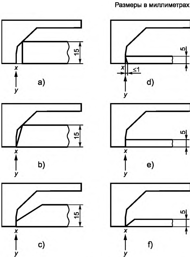
Случаи а) и б) — не соответствуют; случаи с), d), е) и f) — соответствуют (соответствие должно быть проверено требованиями 20.8, используя калибр, представленный на рисунке 23)
