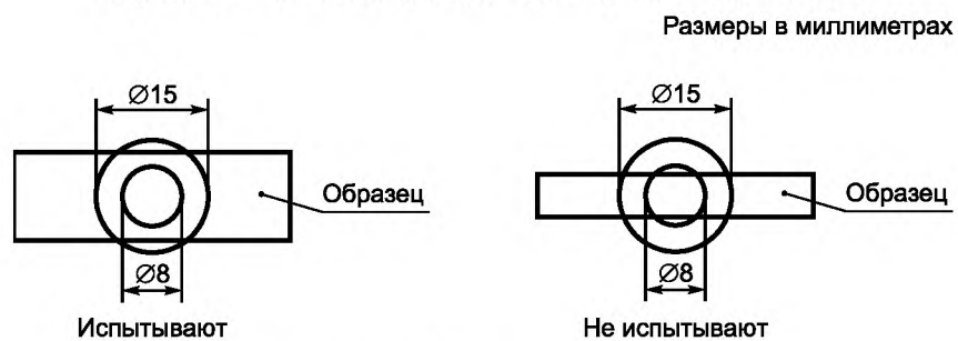
Рисунок 26 — Схема испытания по 24.1.1
