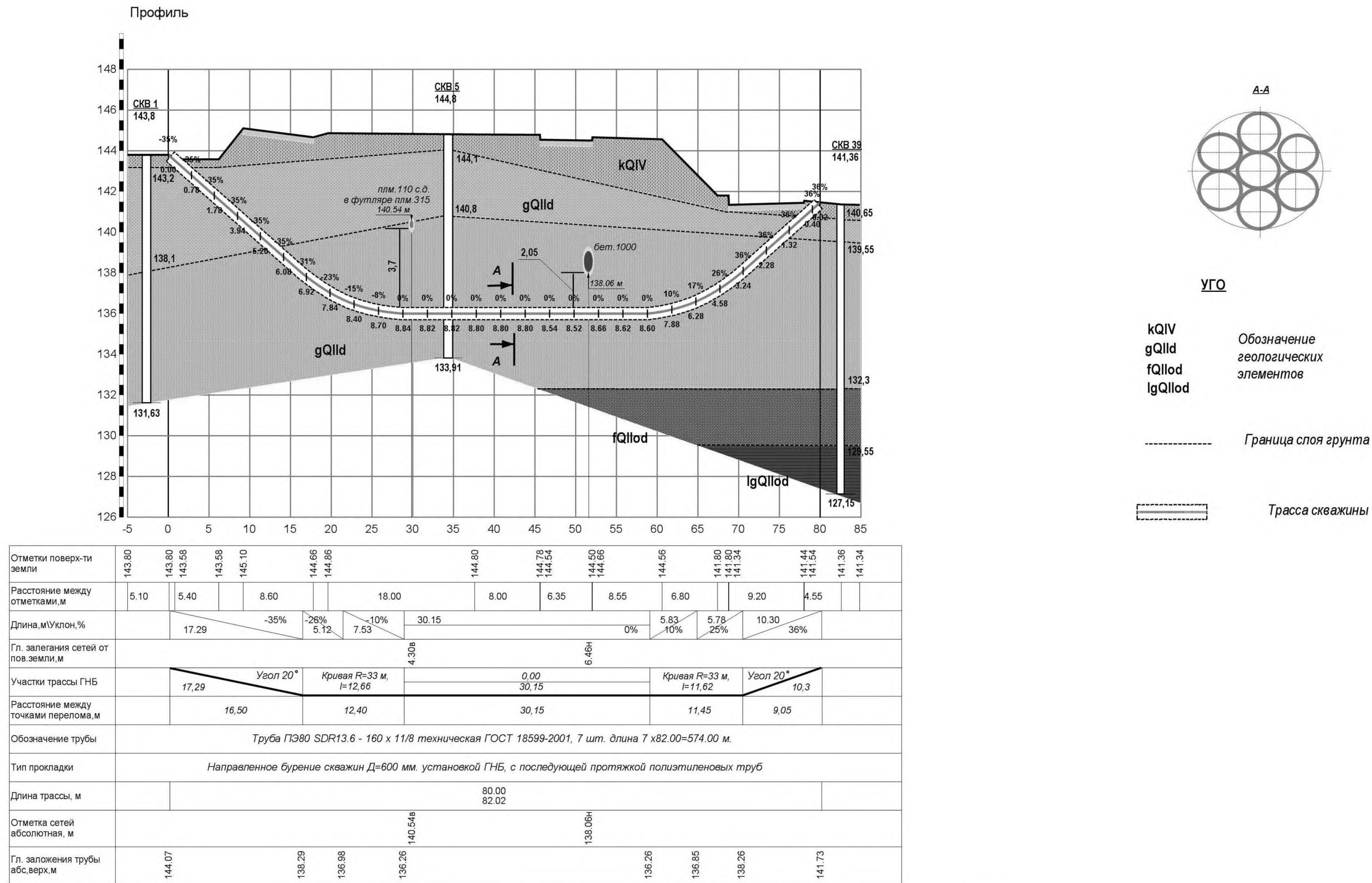
Рисунок 7.1 – Пример построения продольного профиля трассы скважины ГНБ
