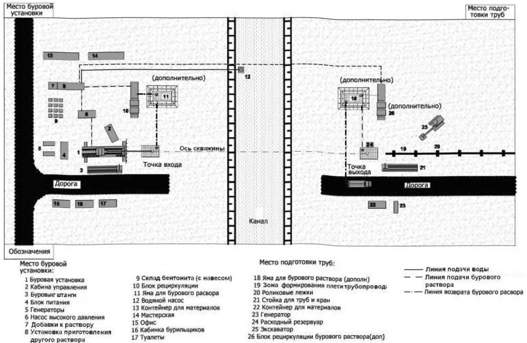
Рисунок 8.1 – Схема расположения оборудования на строительной площадке
