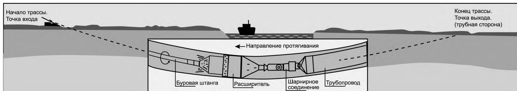
Рисунок 8.6– Сборка буровой колонны для протягивания трубопровода
