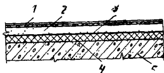
Рис. 2. Конструктивная схема пола с покрытием из линолеума на войлочной основе над неотапливаемыми подвалами и техническими подпольями
