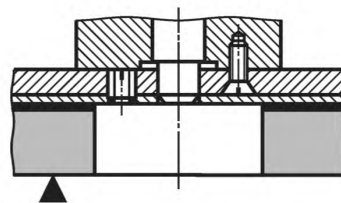
Рисунок 3 — Торцевое шлифование кольцевым кругом
