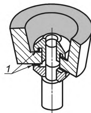
1 — прокладка
