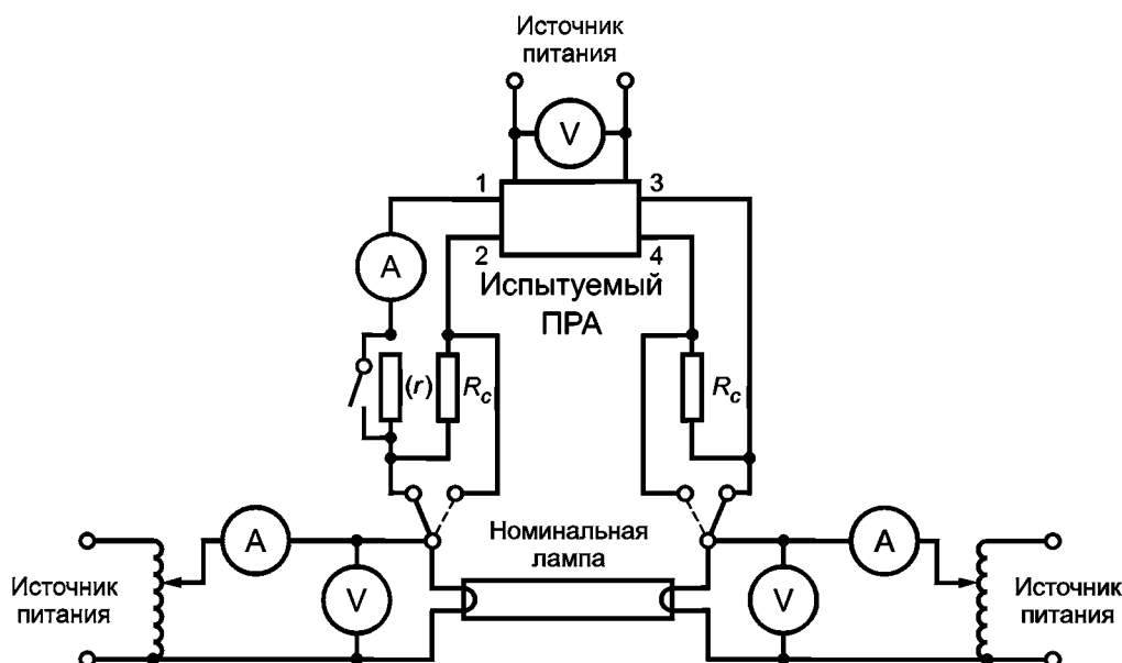
Рисунок A.8 — Схема измерений максимального тока в любом вводе электрода
