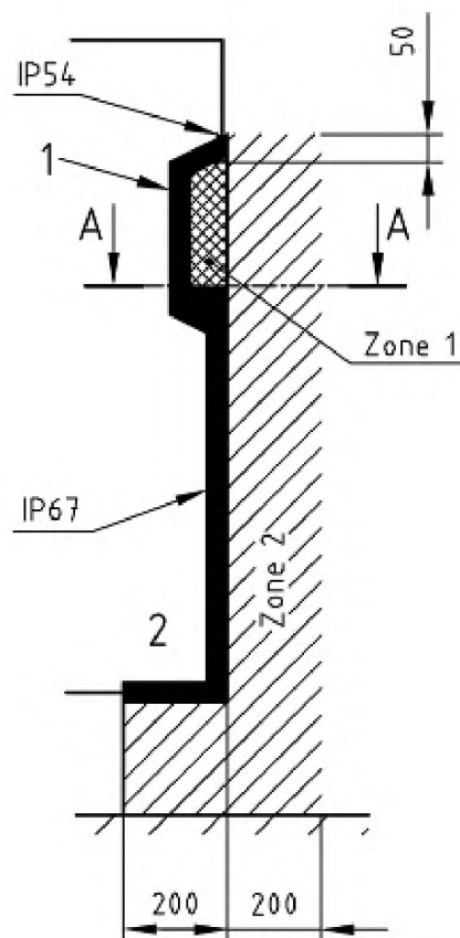
Зона 1: оборудование категории 2 Зона 2: оборудование категории 3 1 – колодка топливораздаточного крана; 2 – взрывобезопасная зона
