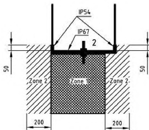
Рисунок А.1 – Тип 1 горизонтальной защиты от проникновения паров топлива
