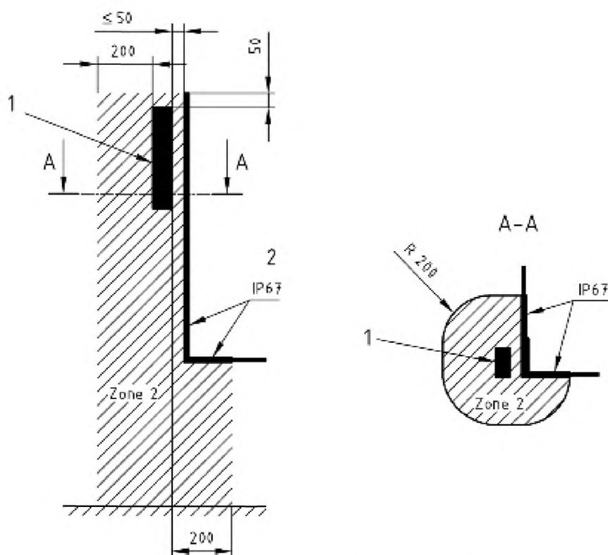
Зона 2: оборудование категории 3 1 – топливораздаточный кран; 2 – взрывобезопасная зона
