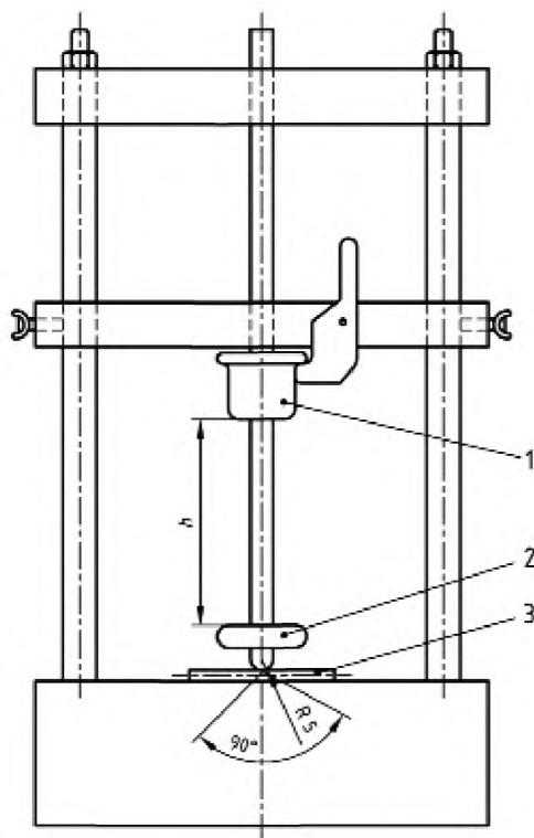
1 – молот; 2 – прокладка из закаленной стали; 3 – образец
