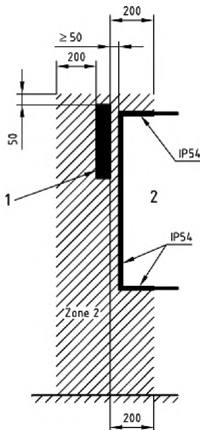
Рисунок 2 – Топливораздаточный кран снаружи кожуха на расстоянии > 50 мм и \leq 200 мм
