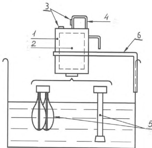
1 – корпус; 2 – двигатель и привод; 3 – переключатель, регулятор частоты вращения двигателя; 4 – рукоятка; 5 – рабочий орган; 6 – опора
