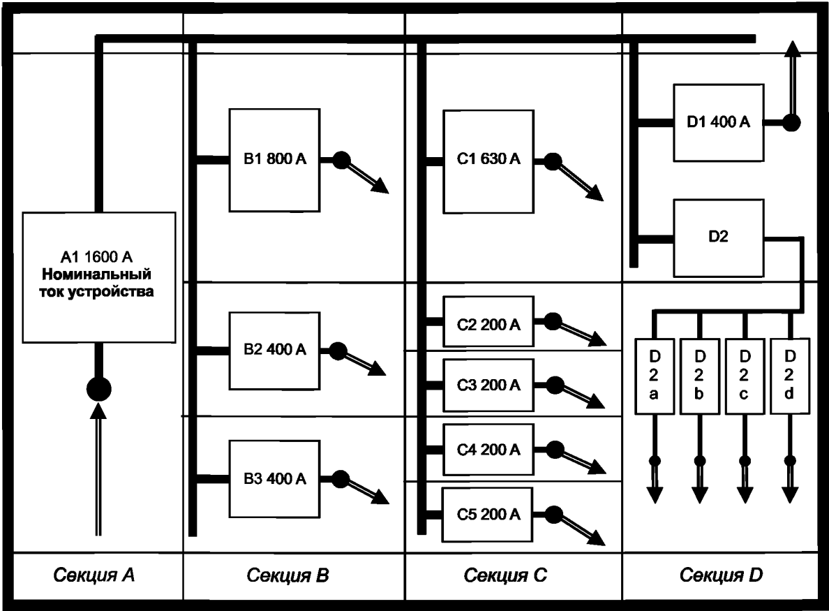
В функциональных блоках показаны номинальные токи ( I_n ) 1) 1) Номинальный ток функциональных блоков (цепей) НКУ не должен превышать номинальный ток устройства.
