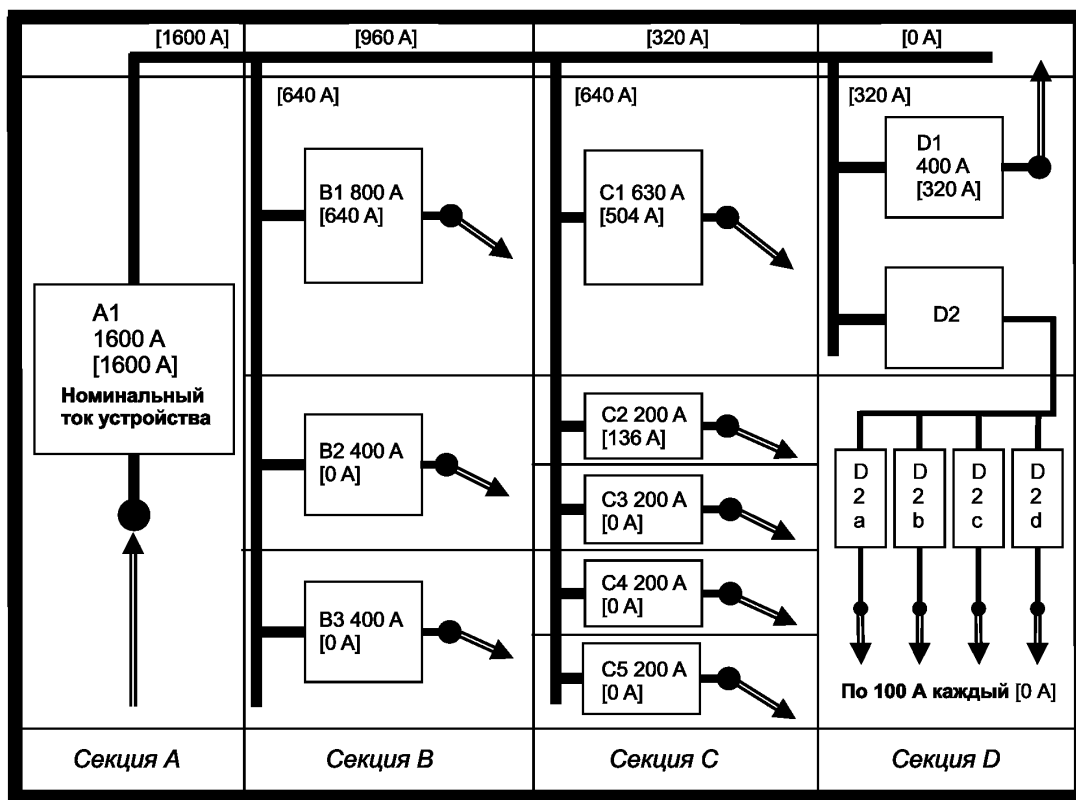
Рисунок Е.3 — Пример 2: Таблица Е.1 — Нагрузка функционального блока для НКУ с номинальным коэффициентом одновременности 0,8
