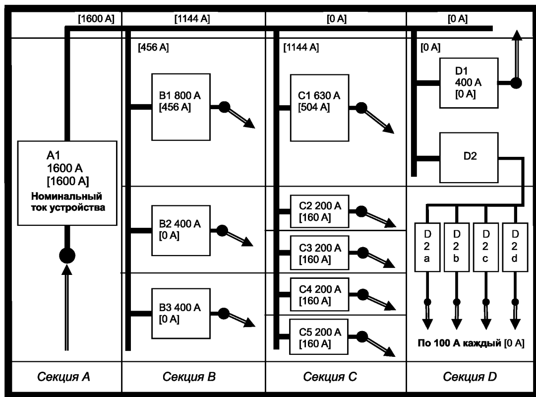
Рисунок Е.4 — Пример 3: Таблица Е.1 — Нагрузка функционального блока для НКУ с номинальным коэффициентом одновременности 0,8
