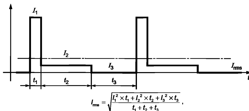
Рисунок Е.6 — Пример среднего расчета теплового эффекта
