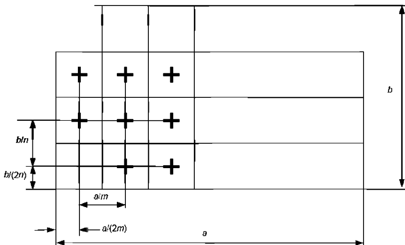
Рисунок 201.101 — Пример сетки для измерения
