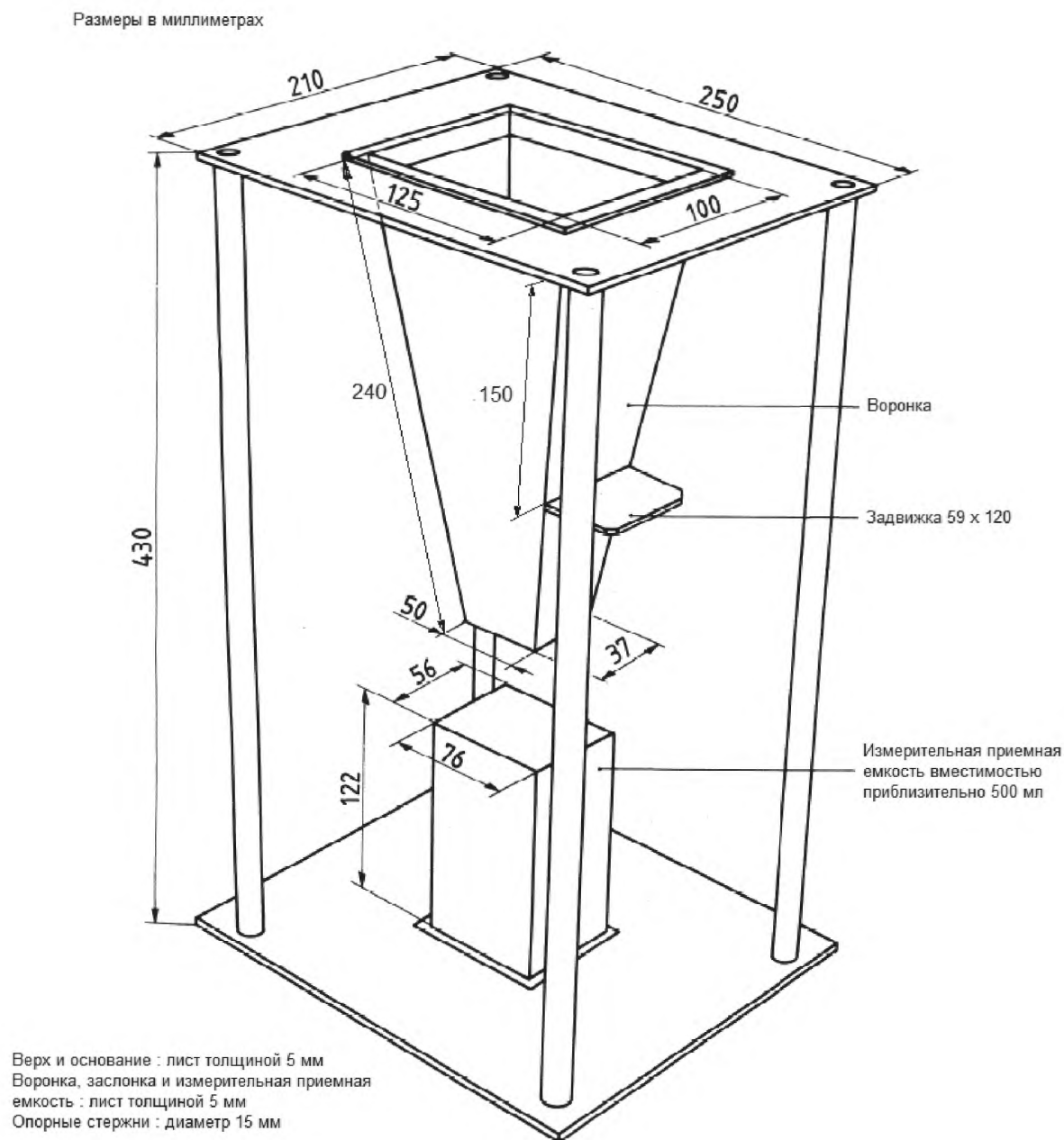
Рисунок 1 – Устройство для определения объемной плотности
