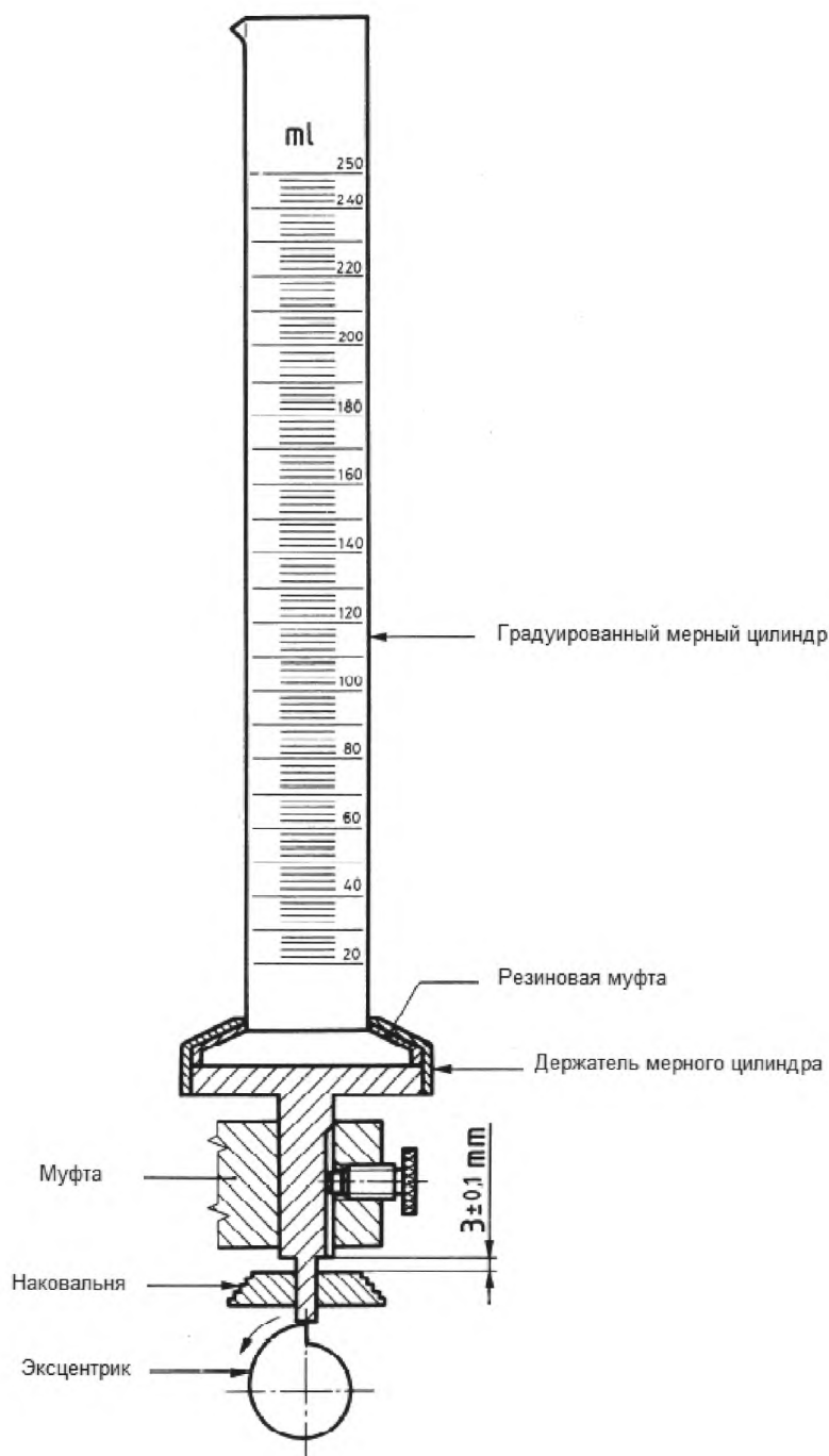
Рисунок 2 – Толчковый измеритель объема
