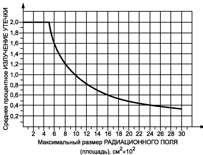
Рисунок 101 — ИЗЛУЧЕНИЕ УТЕЧКИ
