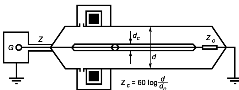
Рисунок 7 — Измерение передаваемых перенапряжений. Схема испытания и элегазовый коммутатор
