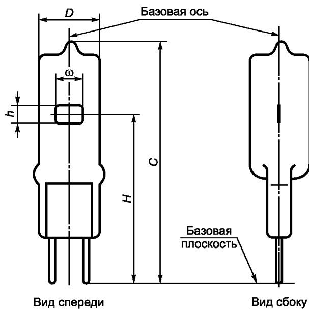
Размеры в миллиметрах
