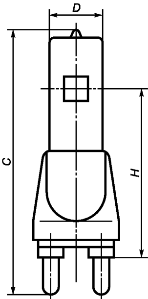
Размеры в миллиметрах
