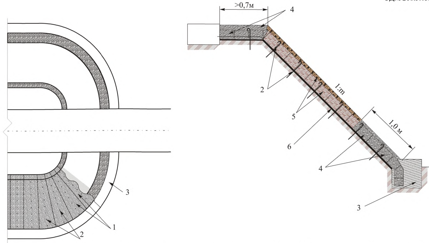
Рисунок 6 – Вариант конструктивного решения укрепления конусов мостов (путепроводов)
