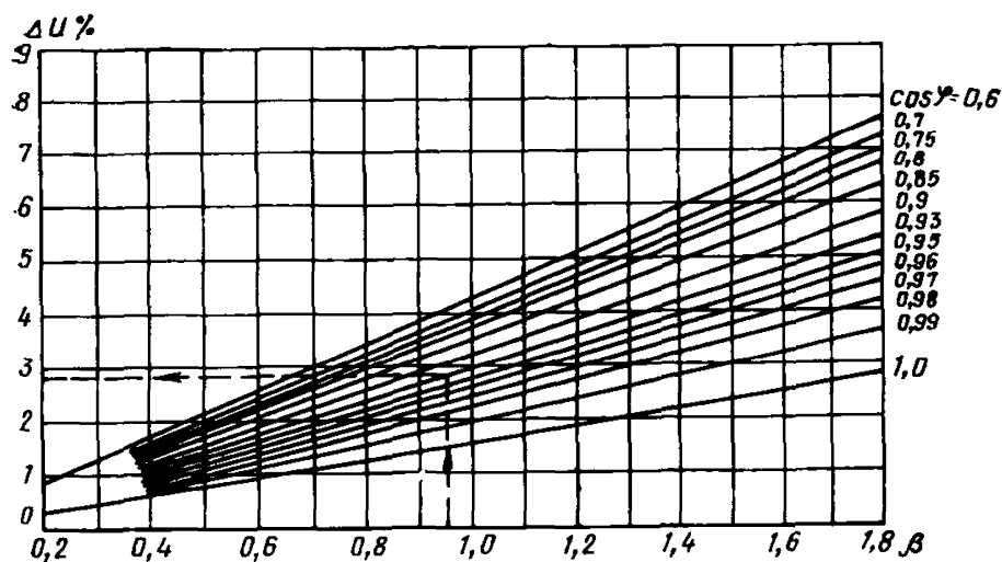
Рис. 33. Графики потерь напряжения в трансформаторе 10(6)/0,4 кВ мощностью 400 кВ·А со схемой соединения обмоток Д/У н -11
