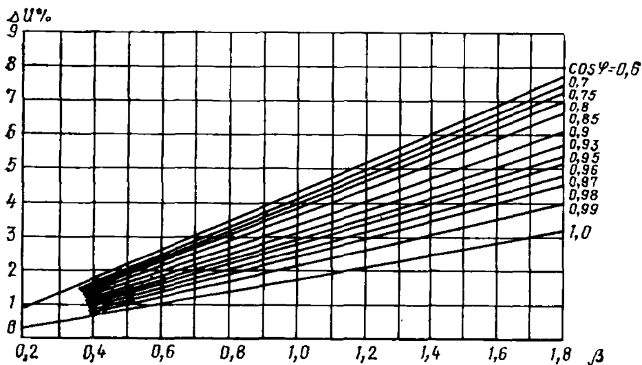
Рис. 34. Графики потерь напряжения в трансформаторе 10(6)/0,4 кВ мощностью 400 кВ·А со схемой соединения обмоток У/У н -0
