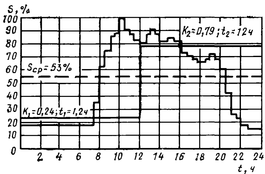
Рис. 6. Графики нагрузки универсама
