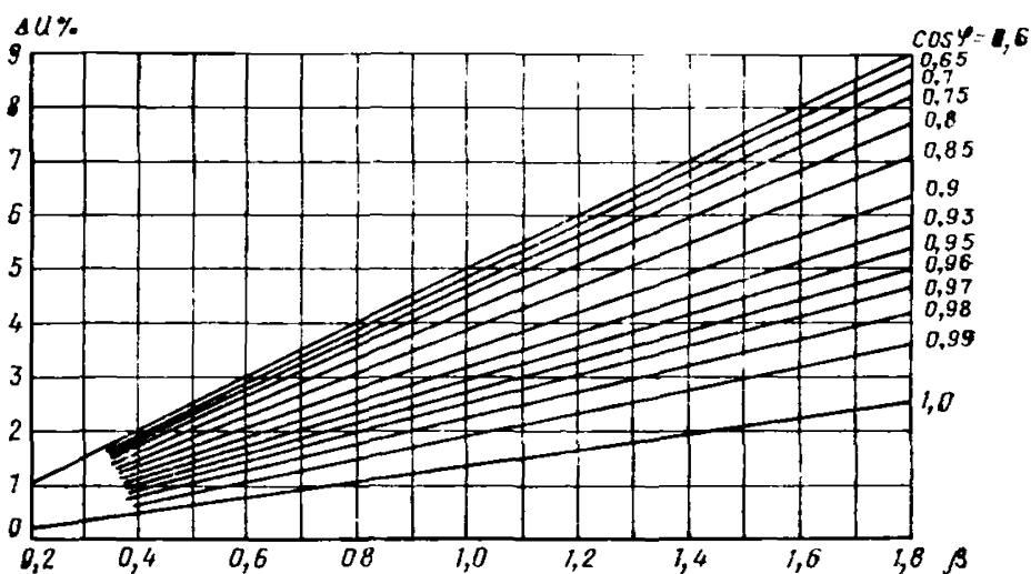
Рис. 36. Графики потерь напряжения в трансформаторе 10(6)/0,4 кВ мощностью 630 кВ·А со схемой соединения обмоток У/У н —0
