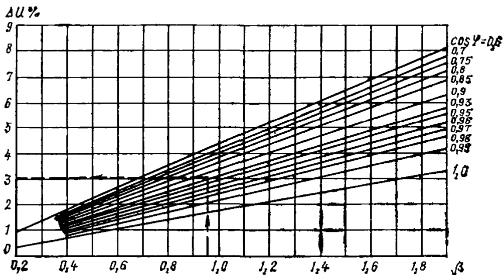
Рис. 31. Графики потерь напряжения в трансформаторе 10(6)/0,4 кВ мощностью 250 кВ·А со схемой соединения обмоток Y/Z_H-11
