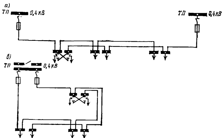
Рис. 16. Двухлучевая схема распределительной сети напряжением 0,4 кВ с двусторонним питанием от: а) разных ТП, б) одной ТП
