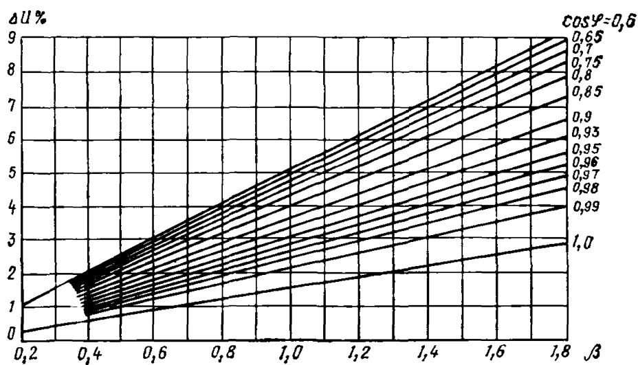
Рис. 35. Графики потерь напряжения в трансформаторе 10(6)/0,4 кВ мощностью 630 кВ·А со схемой соединения обмоток Д/У н —11
