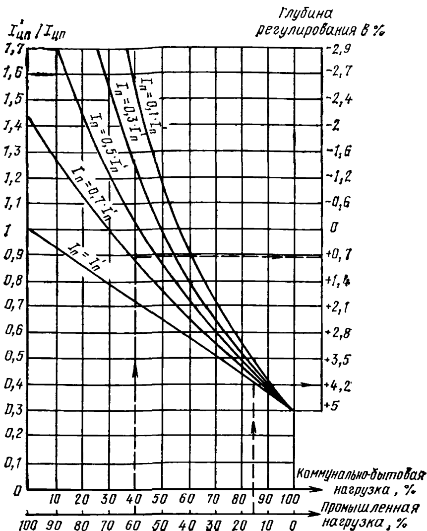
Рис. 39. График зависимости глубины встречного регулирования напряжения от соотношения коммунально-бытовой и промышленной нагрузки на тинах 10(6) кВ ЦП
