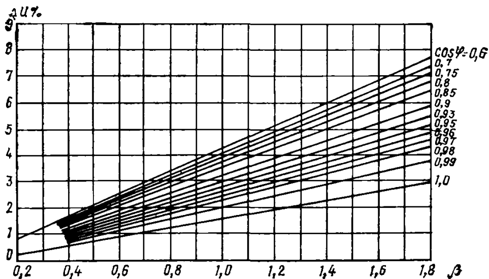
Рис. 32. Графики потерь напряжения в трансформаторе 10(6)/0,4 кВ мощностью 250 кВ·А со схемой соединения обмоток Y/Y_H-0
