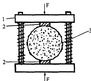
1 – опрессовочная головка; 2 – нагрузочные планки; 3 – образец Рисунок 4 – Опрессовочная головка с нагрузочными планками и образцом для испытаний
