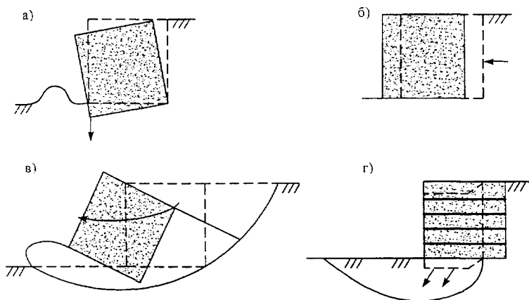
а – опрокидывание; б – горизонтальный сдвиг; в – скольжение по криволинейной поверхности; г – поверхность скольжения, пересекающая сооружение (стрелками показано направление смещения сооружения)
