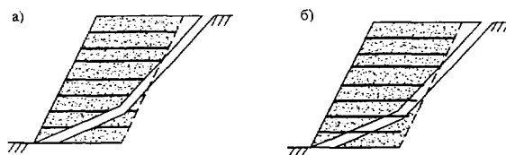
Рисунок 21 – Примеры предельных состояний внутренней местной устойчивости армогрунтовых насыпей армозLEMENTОВ
