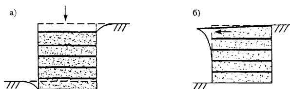
а – осадка основания; б – деформация стены (стрелками показано направление смещения сооружения)
