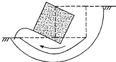
Рисунок 30 – Поверхность скольжения за пределами армогрунтового сооружения
