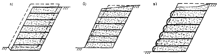
а – осадка основания откоса; б – деформация армозлементов; в – деформация ползучести под влиянием мелких частиц засыпки Рисунок 23 – Примеры состояний предела общей эксплуатационной надежности армогрунтовых насыпей
