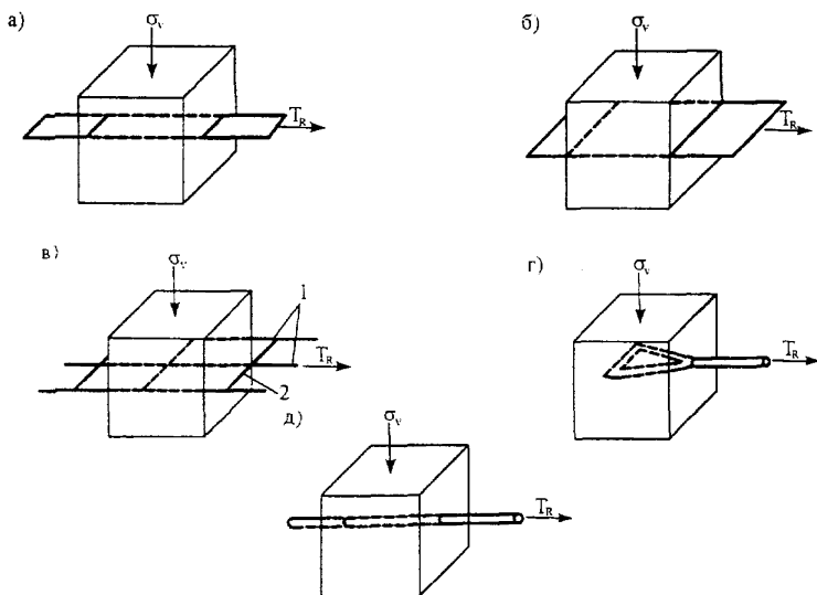
Рисунок 2 – Виды (а, б, в, г, д) армирующих элементов
