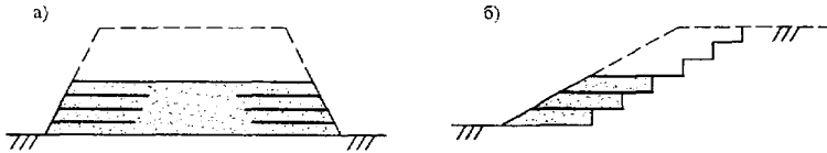
а – армирование новой насыпи; б – восстановление обрушившихся склонов
