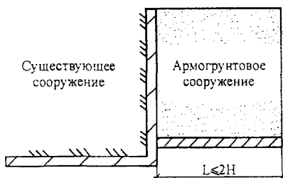
Рисунок 11 – Примыкание к существующему сооружению
