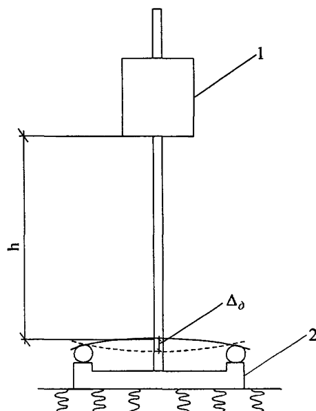
1 — падающий груз; 2 — штамп; h — высота падения груза; \Delta_{\delta} — прогиб упругого элемента под динамической нагрузкой Рисунок 1 — Схема воздействия падающего груза через упругий элемент на дорожную одежду
