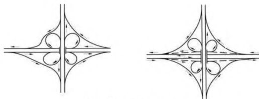
Рис 8.3 Полный клеверный лист
