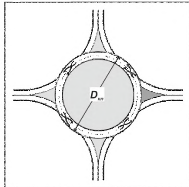
Рис. 7.2 Схемы основных планировочных решений кольцевых пересечений
