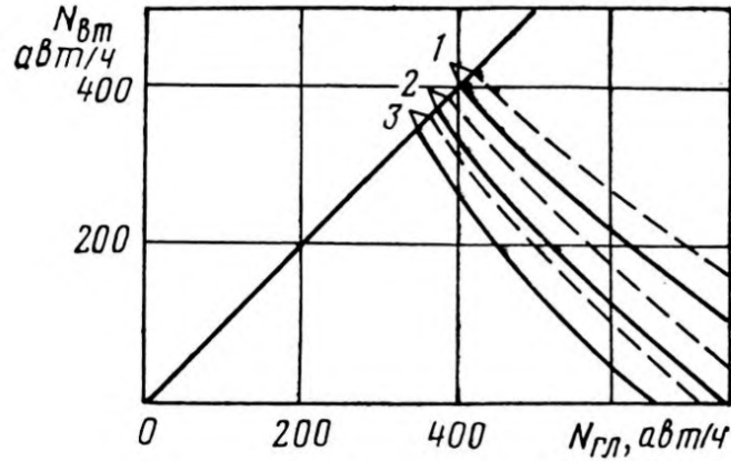
Рисунок А.7. Номограмма для определения пропускной способности нерегулируемых пересечений в одном уровне
