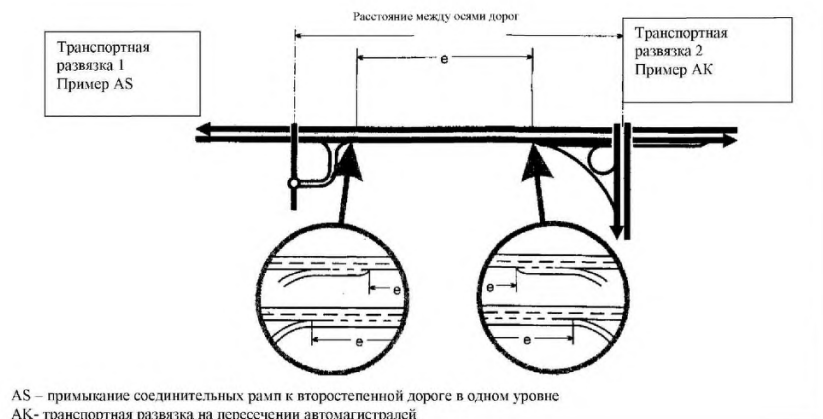
Рис. 5.1 Расстояние e между транспортными развязками.
