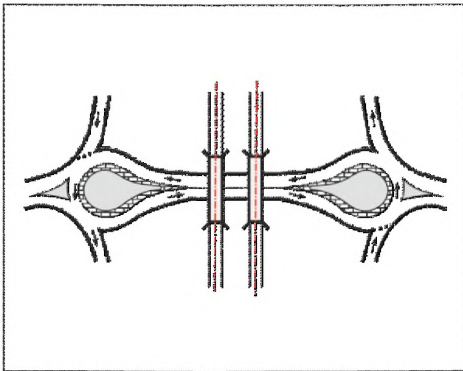
Рис. 7.2 Схемы основных планировочных решений кольцевых пересечений
