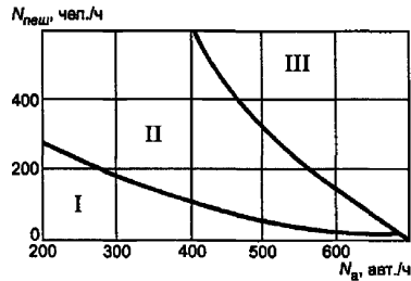
Рис. 12.1 Условия применения пешеходных переходов различных видов: I - нерегулируемые наземные переходы; II – регулируемые наземные переходы; III - внеуличные переходы (надземные и подземные)
