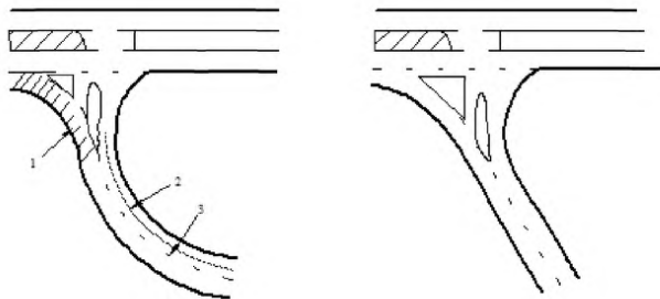
Рис. 6.12 Зрительное перекрытие островками запрещенного направления движения:
