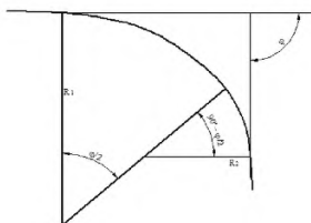
Рис.6.7 Элементы коробовой кривой А – трехзвеньевой, Б – двухзвеньевой
