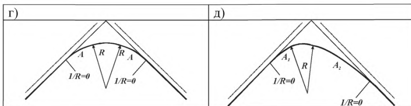
Рис. 6.6 Возможные сопряжения кромок проезжей части:
