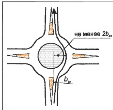
Рис. 7.31 Смещение траектории движения при проезде мини-кольцевого пересечения
