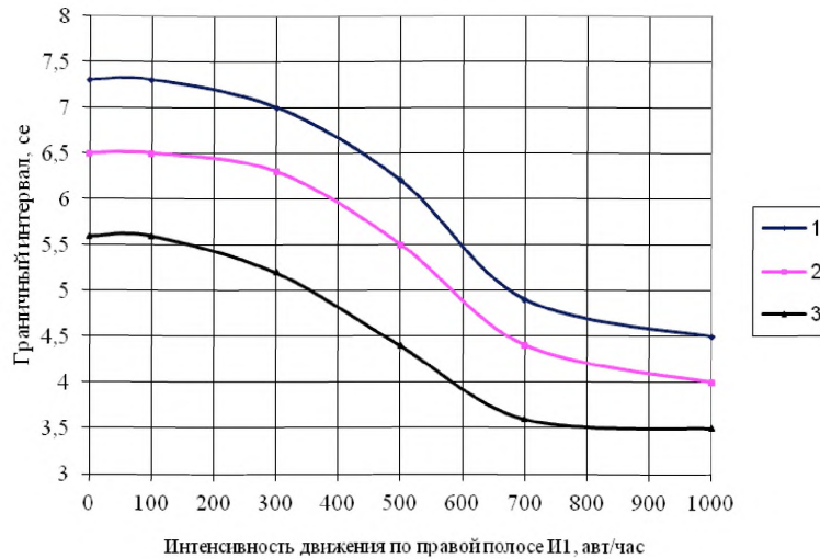
Рис. 1 Зависимость \Delta t_{cp} от интенсивности движения по правой полосе дороги.
