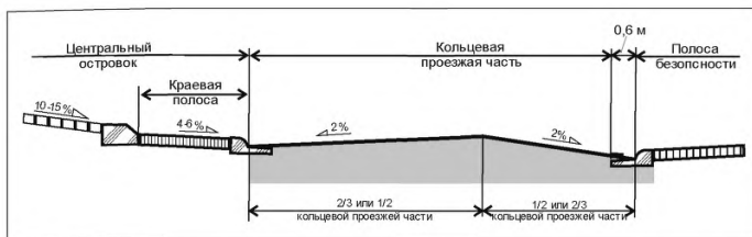
Рис. 7.38 Двухскатный поперечный профиль многополосной кольцевой проезжей части
