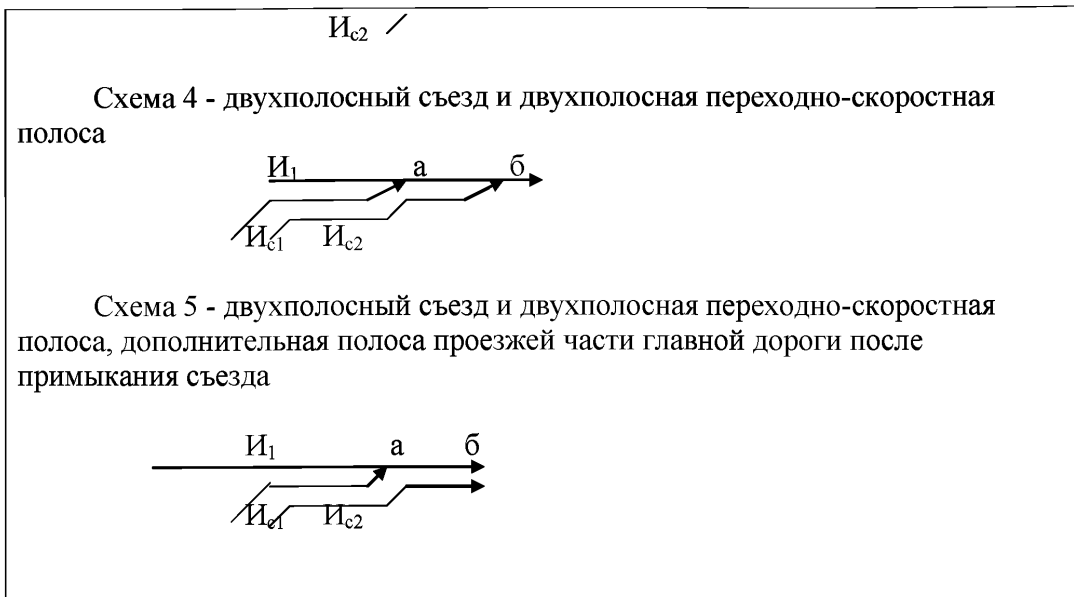
Рис. 2 Схемы слияния транспортных потоков
