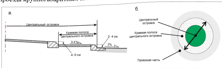
Рис. 7.5 План (а) и поперечный профиль (б) центрального островка с краевой полосой для проезда грузовых автомобилей
