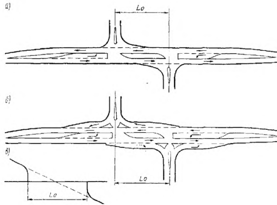
Рис. 6.4 Замена пересечения дорог под острым углом на два примыкания: а - частично канализирование на второстепенной дороге, б - полностью канализированное пересечение, в - схема пересечения.
