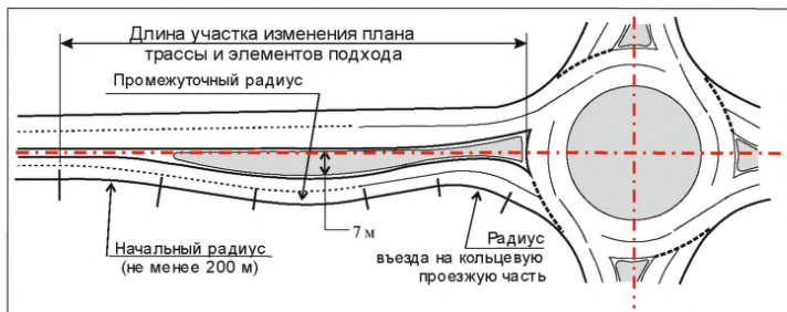
Рис. 7.13 Уширение направляющего островка (центральной разделительной полосы)
