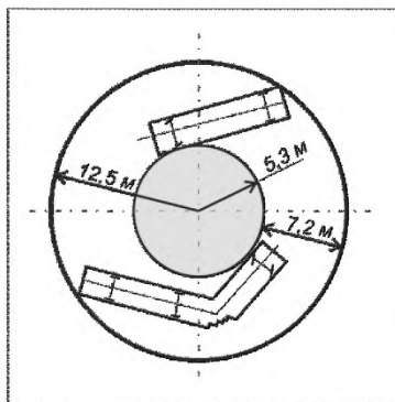
Рис. 7.7 Минимальные размеры поворота сочлененных автобусов
