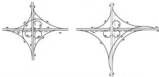
Рис 8.5 Полунаправленные с переплетением
