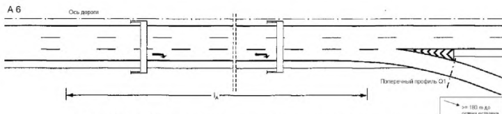
Рис. 9.5 Оформление остроконечного начала съезда
