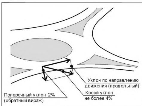
Рис. 7.37 Уклоны кольцевой проезжей части
