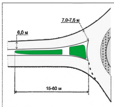
Рис. 7.18 Ширина проезжей части участка въезда однополосного кольцевого пересечения
