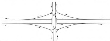
Рис 8.2 Ромбовидное пересечение типа бриллиант
