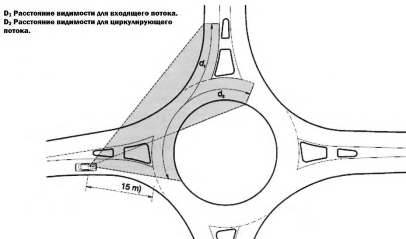
Рис. 15.10. Схема для определения минимального расстояния видимости на пересечении
