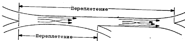
Рис. 10.3 Множественная зона переплетения.
