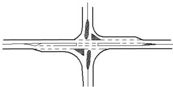
Рис.6.13 Выделение островков на проезжей части разметкой
