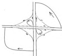
Рис 10.6 б. Развязка типа» клеверный лист» разнесенными съездами
