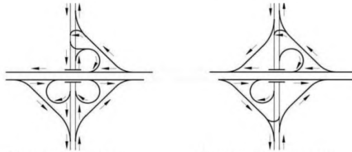
Рис 8.4 Неполный клеверный лист
