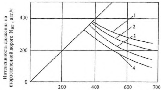
Рисунок А.8. Номограмма для определения практической пропускной способности пересечений в одном уровне.
