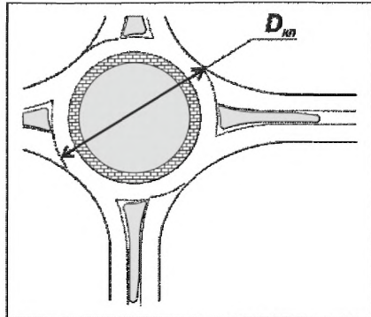
г - мини-кольцевое пересечение
