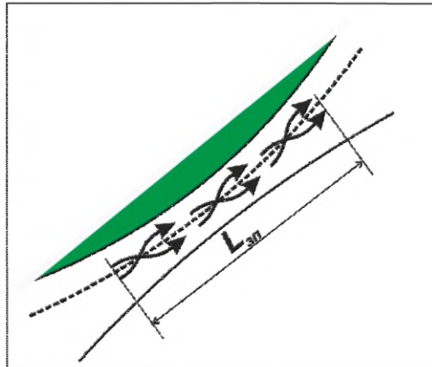
Рис. 7.20 Зона переплетения на кольцевой проезжей части ( L_{зп} )
