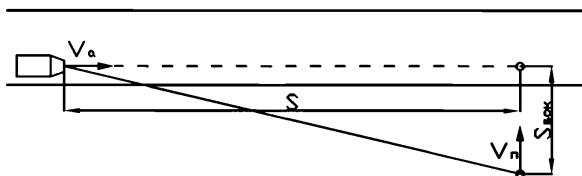
Рис.15.11. Минимальное расстояние боковой видимости у пешеходного перехода
