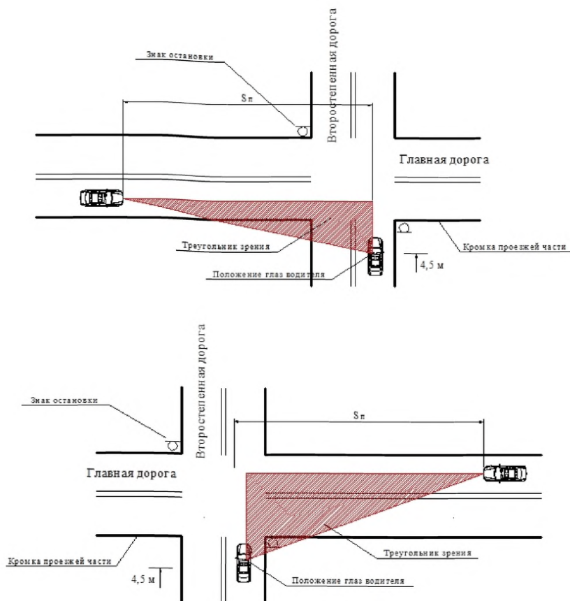
Рис. 15.3 Минимальной расстояние видимости для остановки S на нерегулируемом перекрестке.
