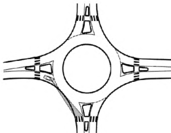
Рис. 15.7 Минимальное расстояние видимости до пешеходного перехода на выезде с кольцевого пересечения
