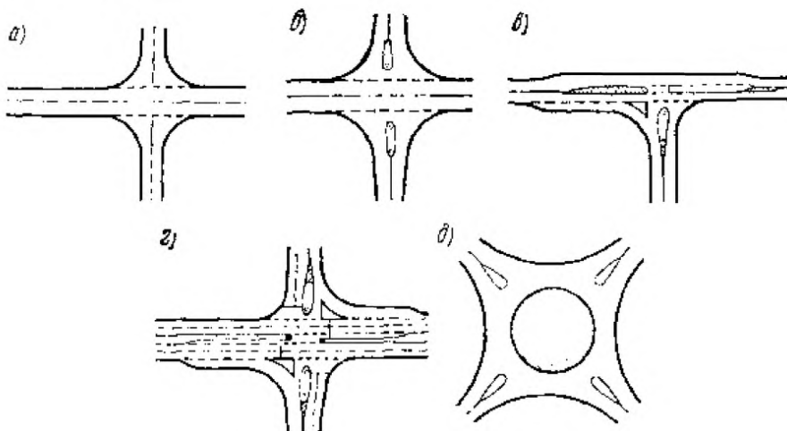
Рис. 6.1 Типы пересечений в одном уровне:
