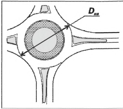
в - кольцевые пересечения большого диаметра ( D_{кп} = 40 - 60 м)
