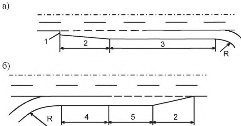
Рис. 9.1 Основные элементы переходно-скоростной полосы
