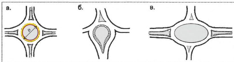
Рис. 7.3 Центральные островки круглой (а), каплеобразной (б) и овальной (в) формы
