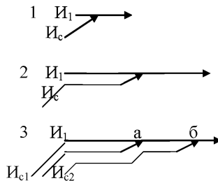
Рис. 10.1 Схемы слияния транспортных потоков.
