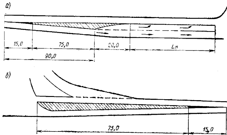
Рис. 6.8, а, б. Разделительные островки на главной дороге:
