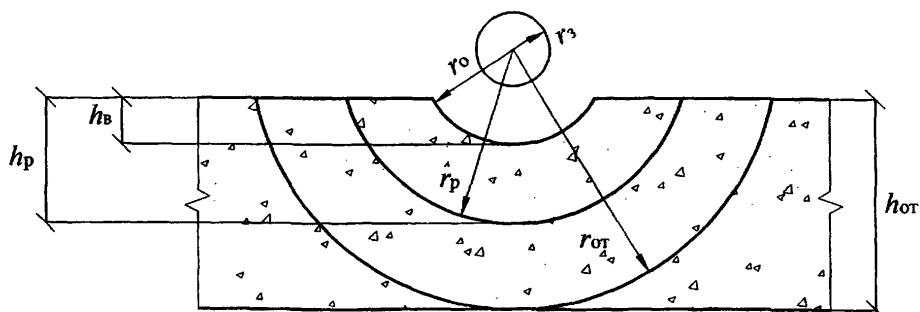
Рисунок Б.2 – Области разрушения преграды при взрыве
