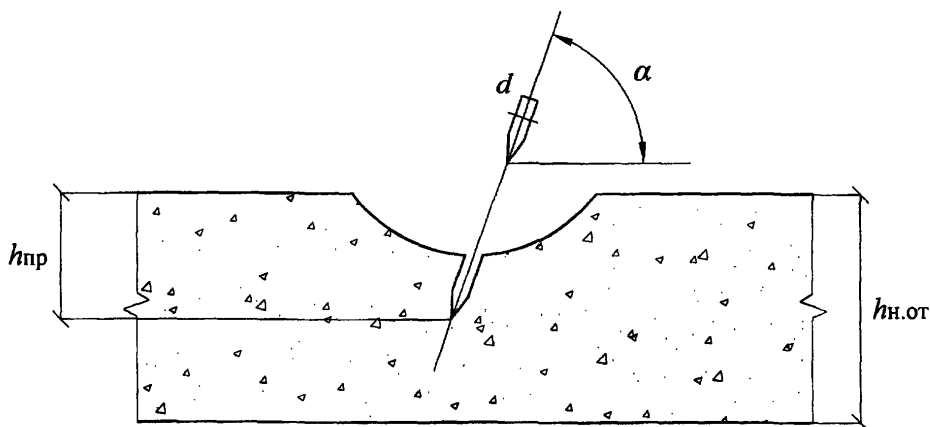
Рисунок Б.1 – Области разрушения преграды при ударе
