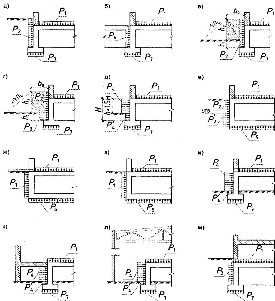
Рисунок 7.1 – Схемы приложения динамических нагрузок на конструкции убежищ
