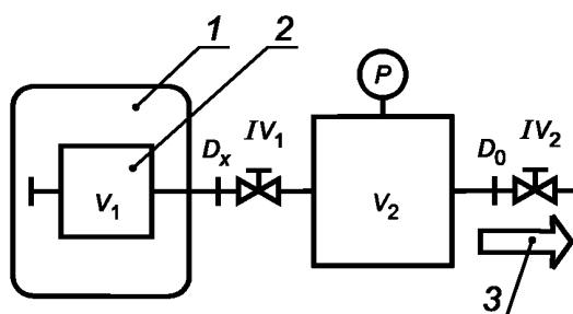
1 — система, заполненная гелием; 2 — испытываемая система; 3 — выход
