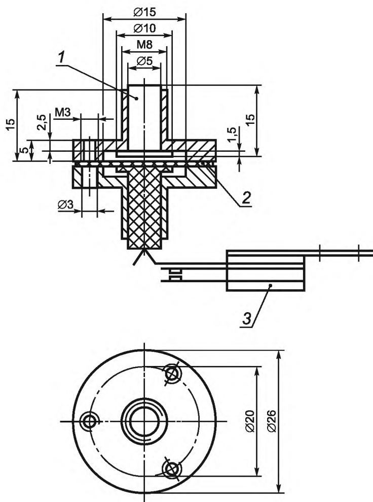
Рисунок 5 — Датчик давления
