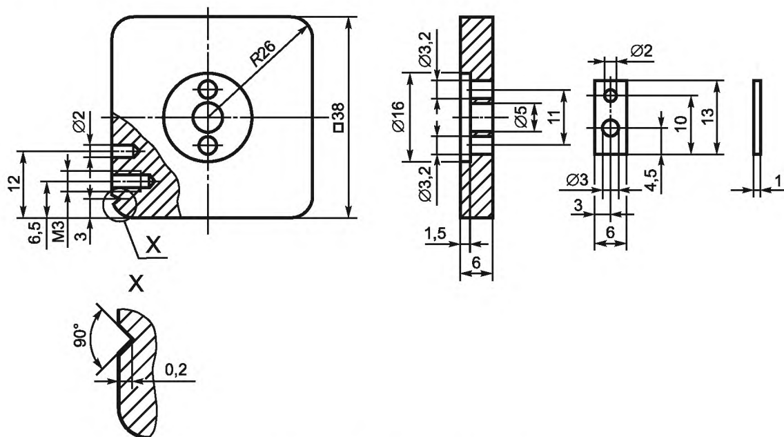
Рисунок 4 — Держатель проволочек
