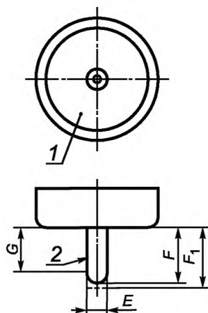
1 – изоляционный материал (вид произвольный); 2 – полированная поверхность для припайки
