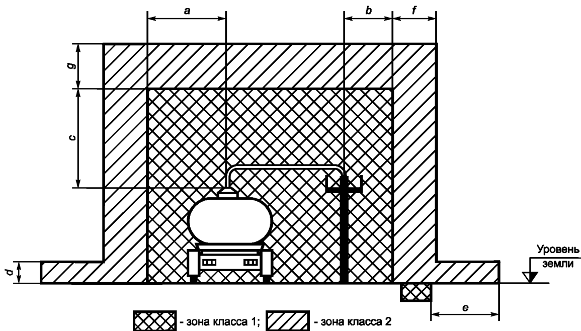
Пример № 9 Установка для заправки бензином автоцистерн, располагаемая снаружи, заполнение которой производится сверху
