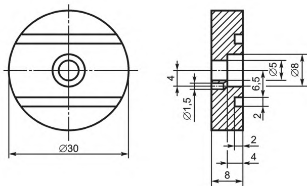
Рисунок Б.2 — Кадмиевый контактный диск
