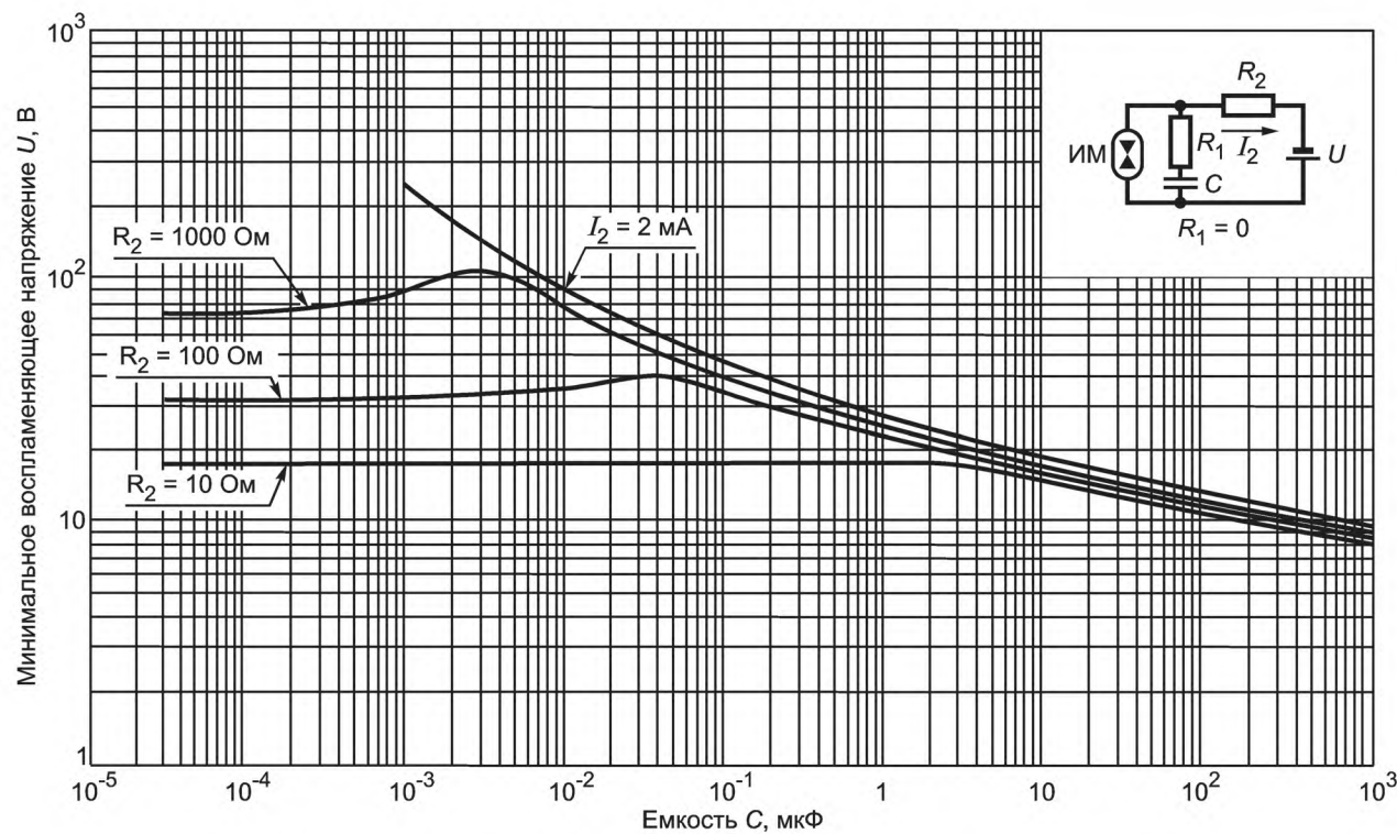
Рисунок А.12 — Минимальное воспламеняющее напряжение в активизированной взрывоопасной водородно-кислородной смеси (81 % H_2 + 19 % O_2 ) для емкостных цепей подгруппы IIA при R_1 = 0 Ом
