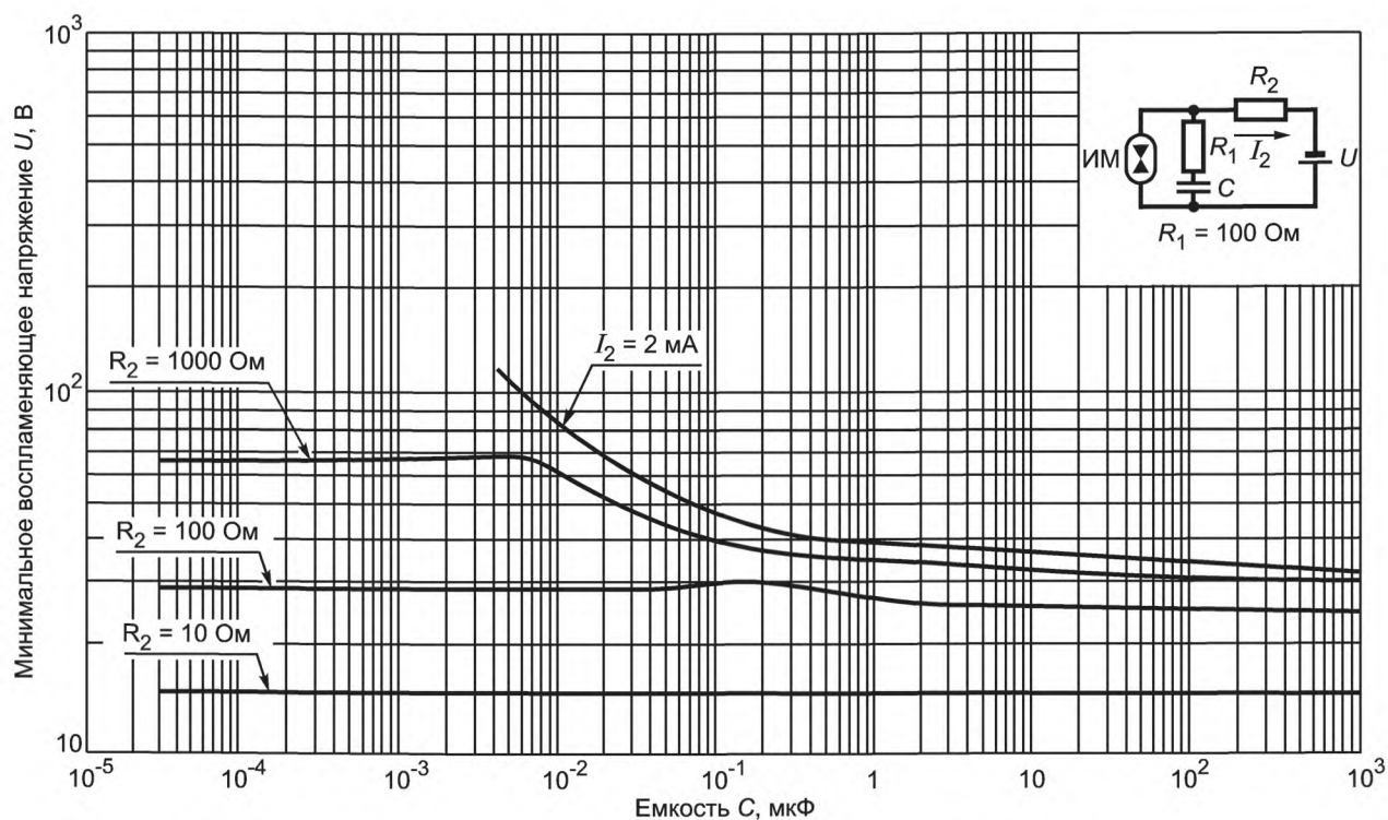
Рисунок А.18 — Минимальное воспламеняющее напряжение в активизированной взрывоопасной водородно-кислородной смеси (75 % \text{H}_2 + 25 % \text{O}_2 ) для емкостных цепей подгруппы IIB при R_1 = 100 \text{ Ом}
