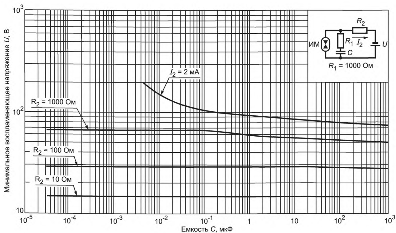
Рисунок А.19 — Минимальное воспламеняющее напряжение в активизированной взрывоопасной водородно-кислородной смеси (75 % \text{H}_2 + 25 % \text{O}_2 ) для емкостных цепей подгруппы IIB при R_1 = 1000 \text{ Ом}
