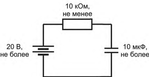
Рисунок А.24 — Простая емкостная цепь
