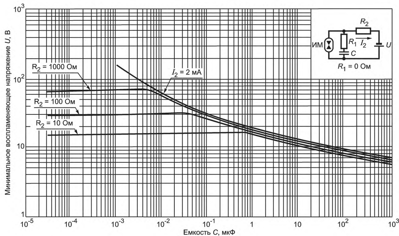
Рисунок А.16 — Минимальное воспламеняющее напряжение в активизированной взрывоопасной водородно-кислородной смеси (75 % H_2 + 25 % O_2 ) для емкостных цепей подгруппы IIB при R_1 = 0 \text{ Ом}
