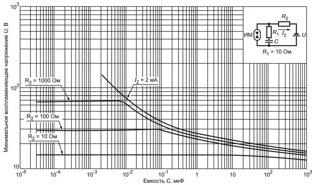
Рисунок А.17 — Минимальное воспламеняющее напряжение в активизированной взрывоопасной водородно-кислородной смеси (75 % H_2 + 25 % O_2 ) для емкостных цепей подгруппы IIB при R_1 = 10 \text{ Ом}
