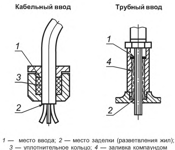
Рисунок 2 — Место ввода и заделки кабеля (разветвления жил)
