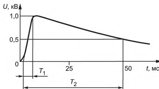
Рисунок 6 — Импульс высокого напряжения
