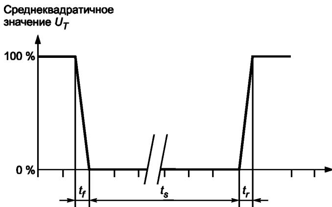
t_f — время нарастания напряжения; t_r — время понижения напряжения; t_s — время выдержки на пониженном напряжении
