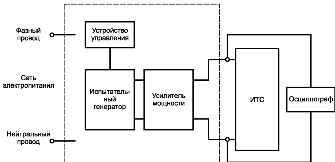
б) Схема испытаний с использованием усилителя мощности
