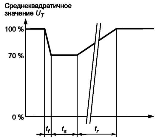
t_f — время понижения напряжения; t_r — время нарастания напряжения; t_s — время выдержки на пониженном напряжении
