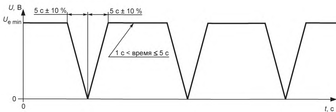
Рисунок 9 — Испытание на быстрое изменение напряжения питания
