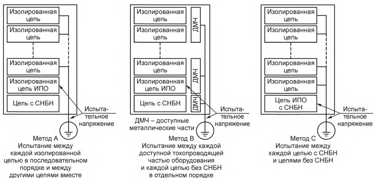
Рисунок 13 — Методы испытания на электрическую прочность диэлектрика
