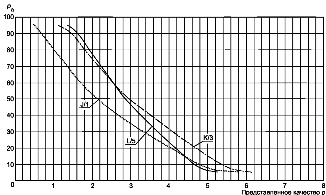
Рисунок 6 — Кривые рабочих характеристик ОС (PX) для планов однократного выборочного контроля на некритичные несоответствия, процедура В
