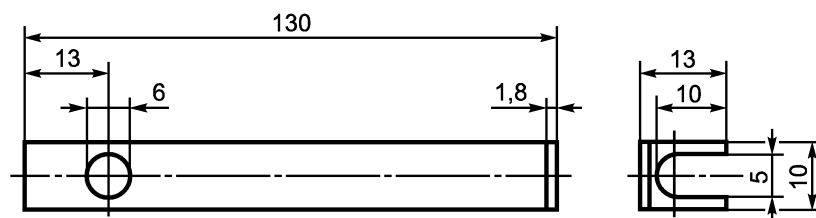
Рисунок 3 — Испытательная жила (см. 11.2)
