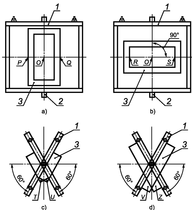
1 — монтажная опора; 2 — шарнир; 3 — образец
