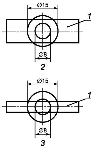
Рисунок 21 — Испытания раскаленной проволокой (см. раздел 18)
