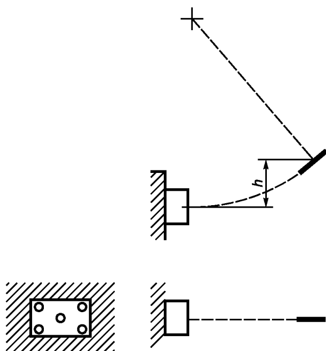
Рисунок 8 — Установка для испытаний на воздействие ударных нагрузок при низкой температуре (см. 15.1)
