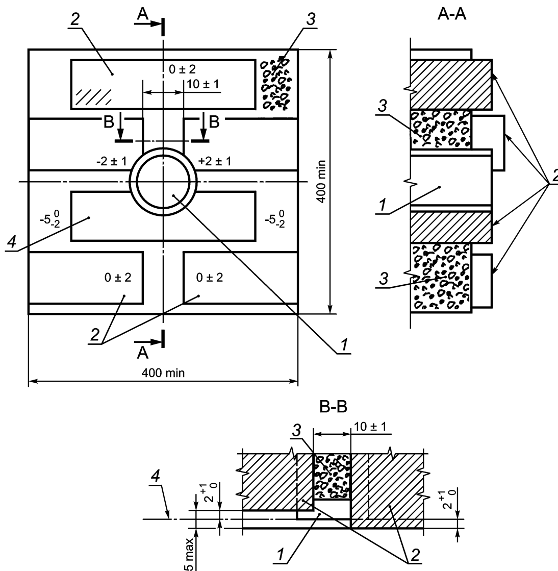
Рисунок 4 — Определение объема (см. 12.12.5)
