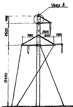
Анкерно-угловая железобетонная одноопелная опора на оттяжках
