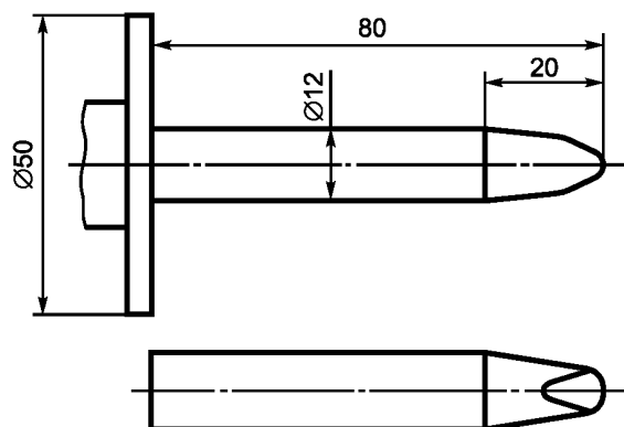
Рисунок В.1 — Жесткий испытательный палец (испытательный щуп по стандартам государств )
