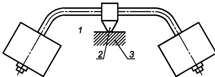
1 — испытываемая часть; 2 — сферическая часть устройства; 3 — опора
