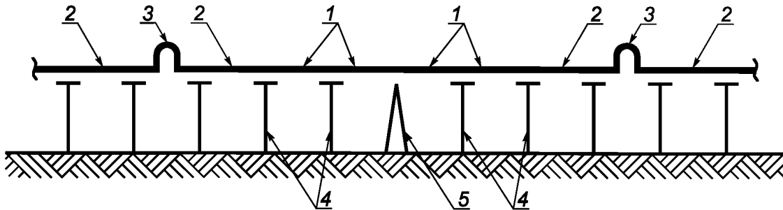
Рисунок 1 — Конструкции опор надземного перехода газопровода
