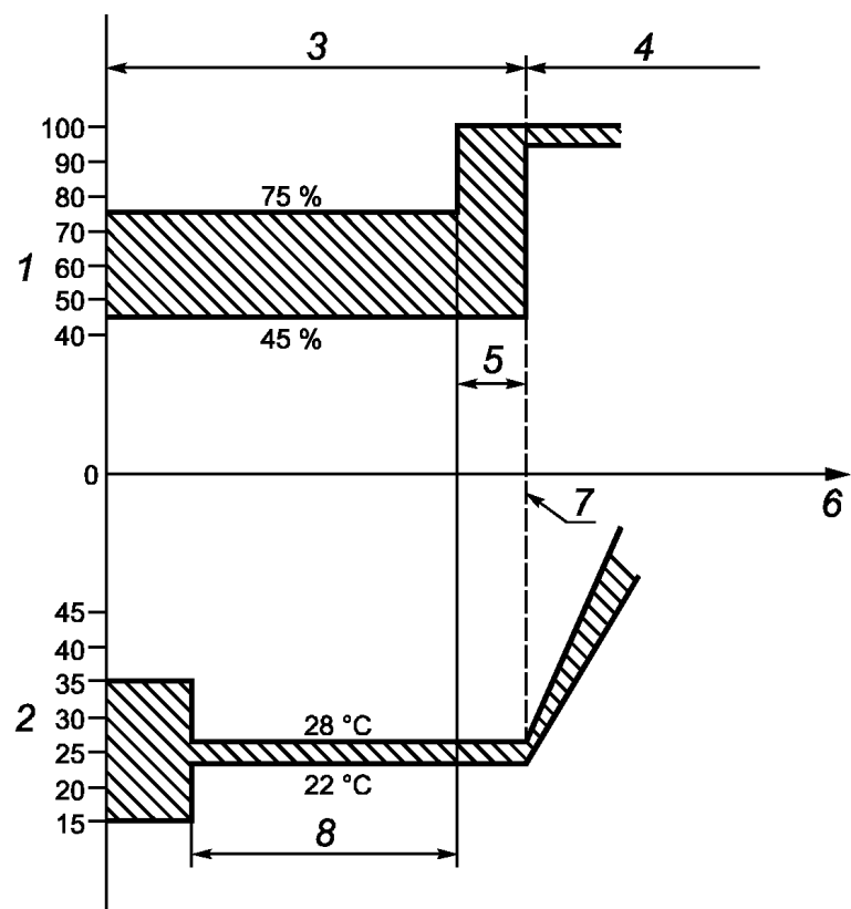
1 — относительная влажность, %; 2 — температура окружающего воздуха, °C; 3 — период стабилизации; 4 — первый цикл; 5 — время, требуемое для достижения 95 — 100 % относительной влажности (не превышающее 1 ч); 6 — время; 7 — начало первого цикла; 8 — время, требуемое испытываемому образцу, чтобы достичь температурной стабильности
