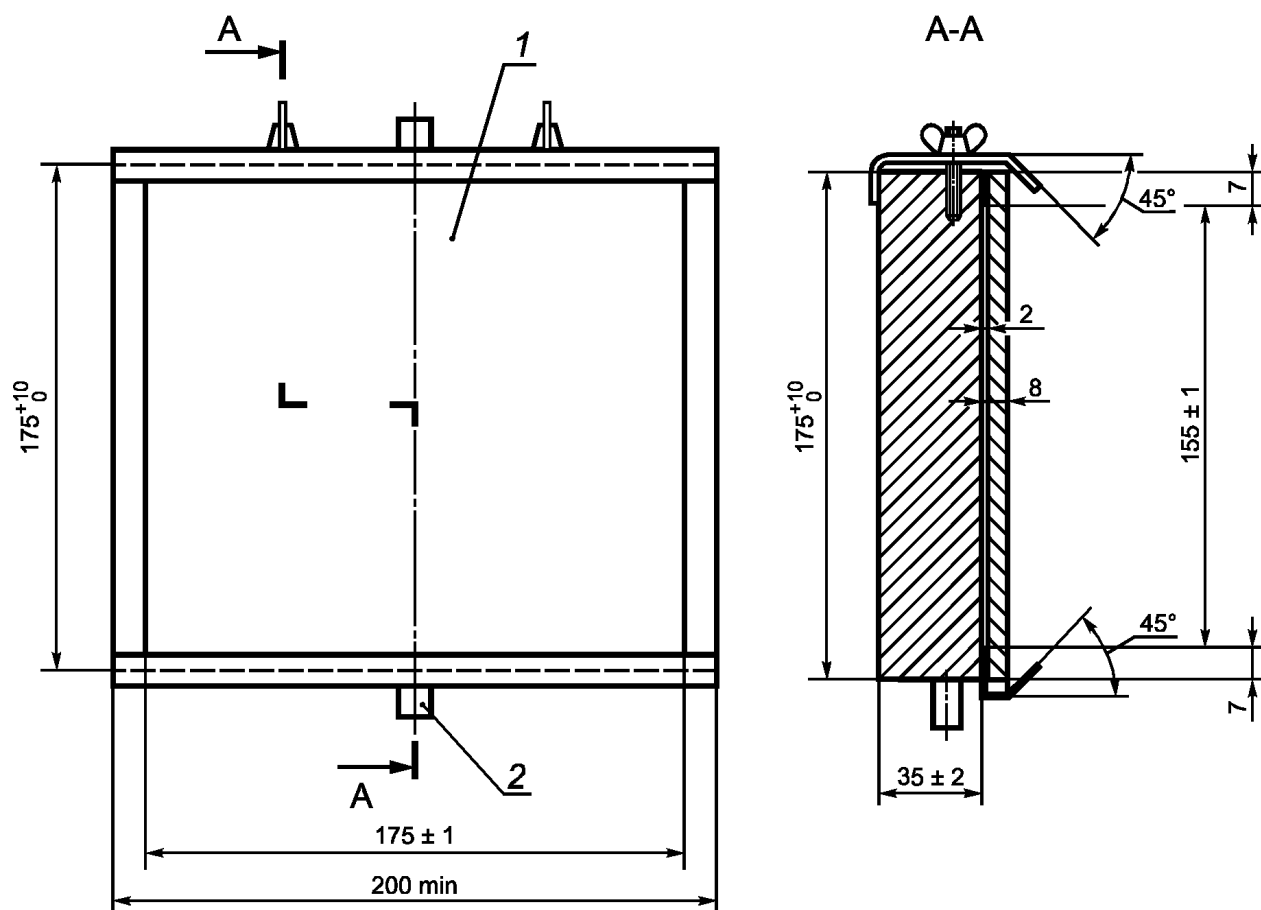
1 — лист фанеры; 2 — шарнир
