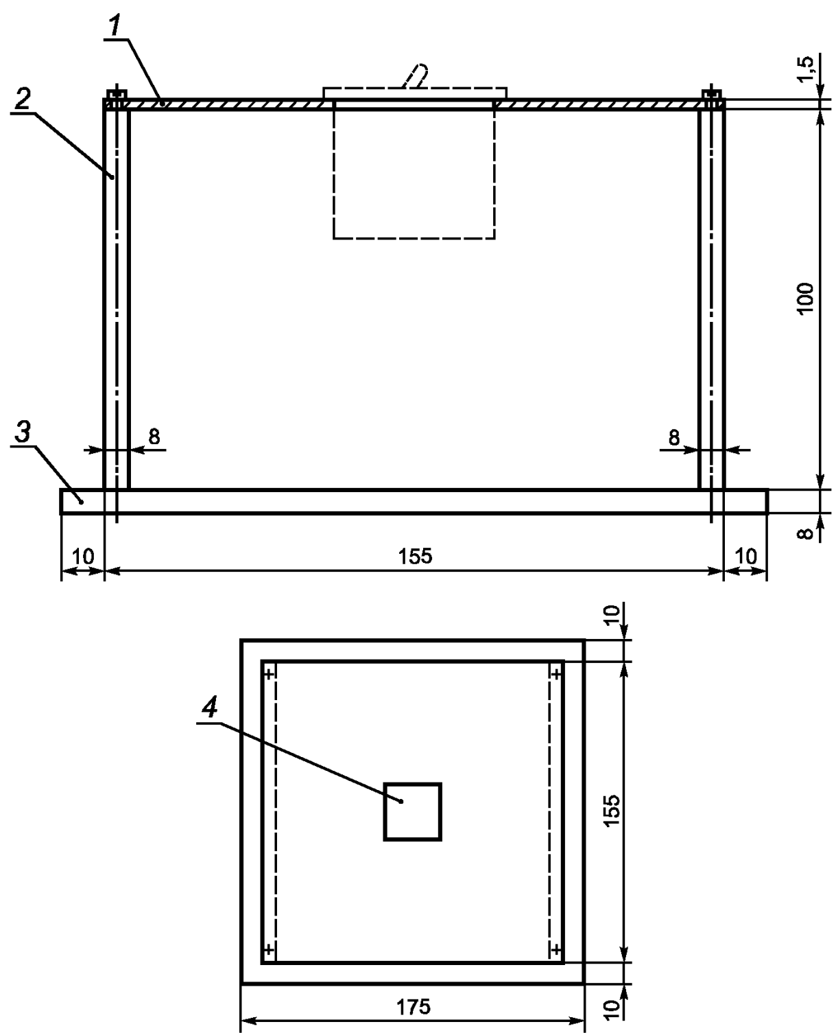
1 — съемная стальная пластина толщиной 1,5 мм; 2 — алюминиевые пластины толщиной 8 мм; 3 — монтажная пластина; 4 — окно в стальной пластине для ВДТ
