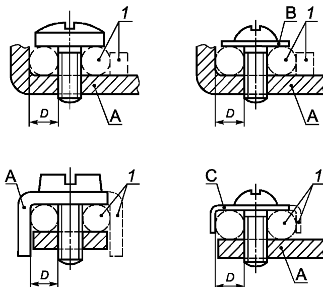
Рисунок IC.2a — Винтовые зажимы
