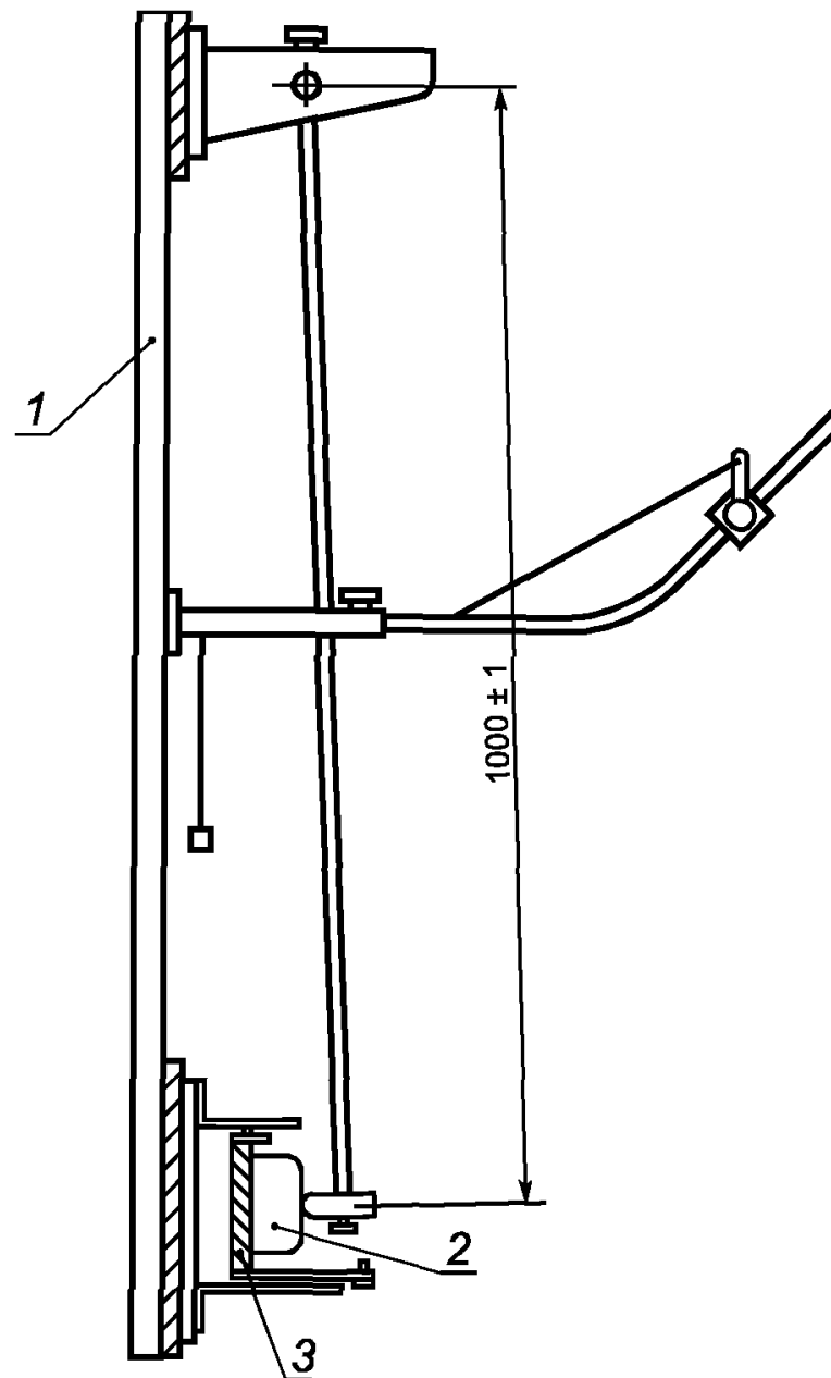
1 — рама; 2 — образец; 3 — монтажная опора
