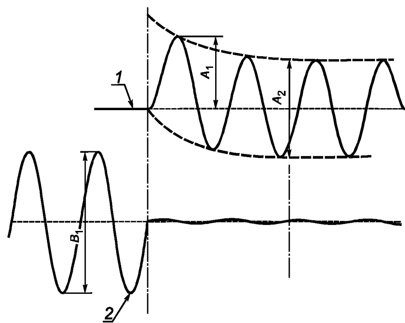
1 — ток; 2 — напряжение
