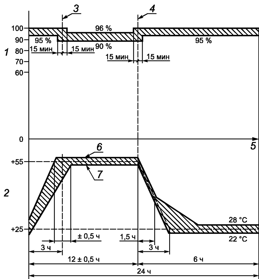
1 — относительная влажность, %; 2 — температура окружающего воздуха, °C; 3 — конец повышения температуры; 4 — начало снижения температуры; 5 — время; 6 — нижнее значение температуры 57 °C; 7 — верхнее значение температуры 53 °C
