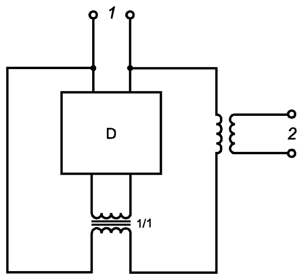
1 — источник напряжения 1,1 U_n ; 2 — источник тока
