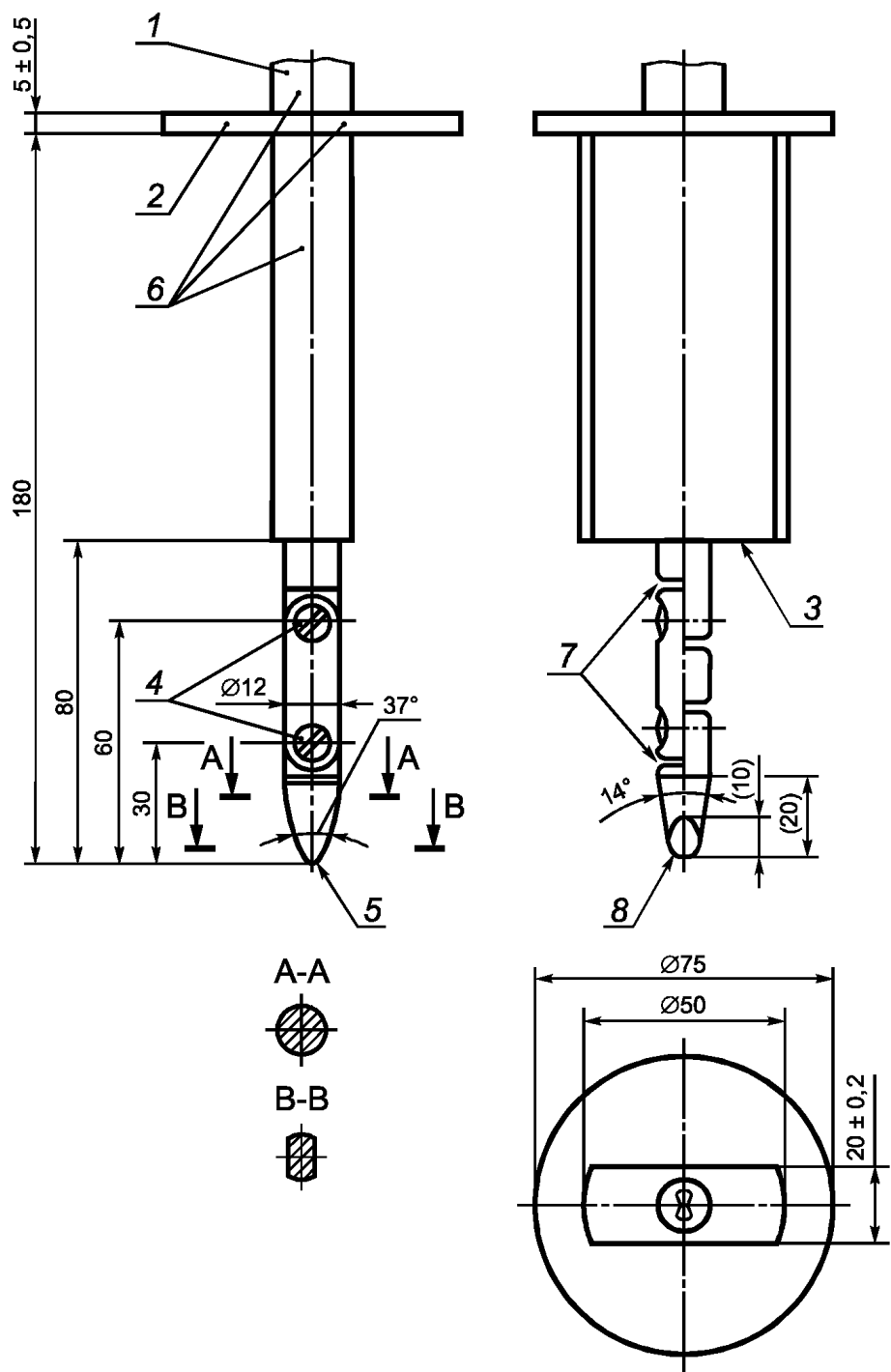
1 — ручка; 2 — защитная шайба; 3 — упорная поверхность; 4 — шарниры; 5 — цилиндр с радиусом R2 \pm 0,05 ; 6 — изоляционный материал; 7 — фаски;
