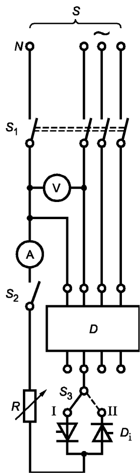
S — источник питания; V — вольтметр; A — амперметр (измерение действующего значения); D — испытуемый ВДТ; D_i — тиристоры; R — переменный резистор; S_1 — выключатель для всех полюсов; S_2 — однополюсный выключатель; S_3 — переключатель на два положения
