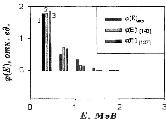
Рис.1. Гистограммы спектров фотонного излучения: 1 – исходный \Phi(E)_{\text{апр}} ( E_{\text{ср}} = 0,567 МэВ), 2 – восстановленный с использованием метода Y.Su ( E_{\text{ср}} = 0,526 МэВ), 3 – восстановленный с использованием метода регуляризации Тихонова А.Н. ( E_{\text{ср}} = 0,512 МэВ)
