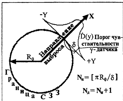
Рис.1. Иллюстрация выбора оптимального количества датчиков АСКРО
