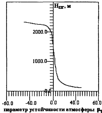
Рис.1. Зависимость высоты пограничного слоя атмосферы от состояния ее устойчивости, характеризующейся параметром \mu_0
