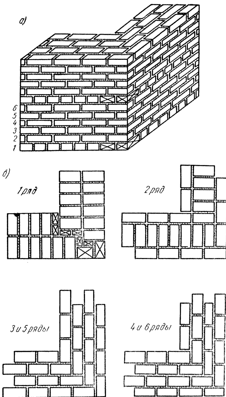
Рис. 2. Многорядная система перевязки a —общий вид кладки угла стены; б —кладка 1, 2, 3, 4, 5, 6-го рядов
